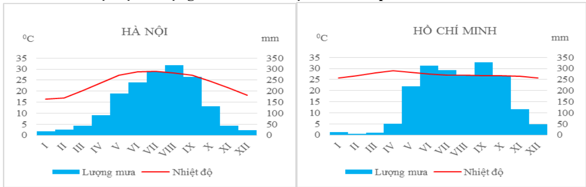
Nhiệt độ và lượng mưa của Hà Nội và Thành phố Hồ Chí Minh
