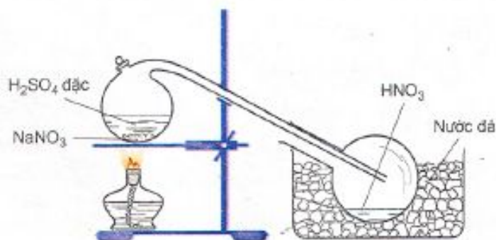
Hình 2.9. Điều chế \text{HNO}_3 trong phòng thí nghiệm
