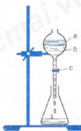
Hình 4.2. Chiết 2 lớp chất lỏng
