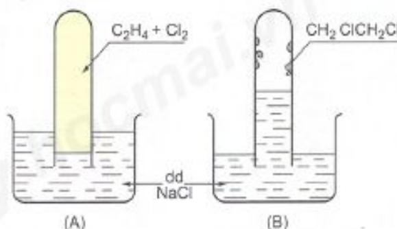
Hình 6.3. Phản ứng của etilen với clo
