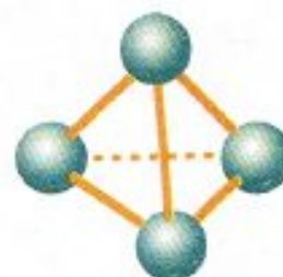
Hình 2.11. Mô hình phân tử P_4
