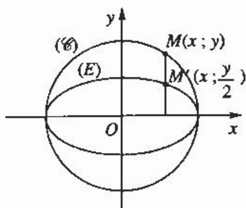
Hình 85. Phép co về trục hoành theo hệ số k = \frac{1}{2} biến đường tròn (C) thành elip (E).
