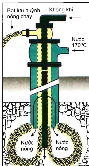
Hình 6.10. Thiết bị khai thác lưu huỳnh (phương pháp Frasch)
