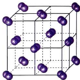
Phân tử I_2
