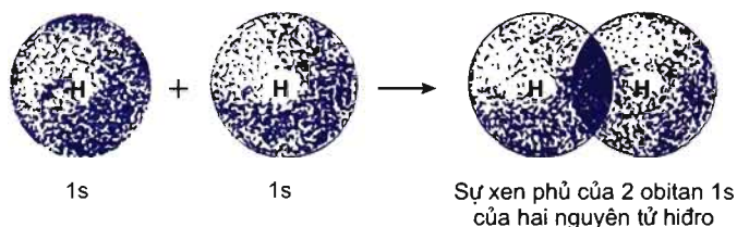
Hình 3.2. Sự hình thành phân tử hydro
