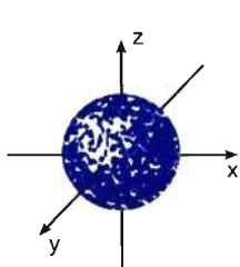
Hình 1.9. Obitan s
