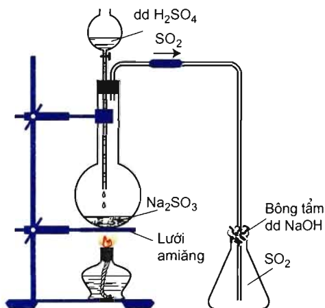
Hình 6.12. Điều chế \text{SO}_2 trong phòng thí nghiệm
