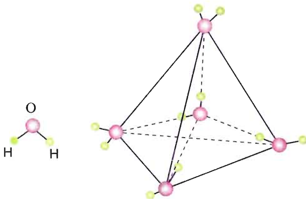
Hình 3.14. Mô hình mạng tinh thể phân tử nước đá
