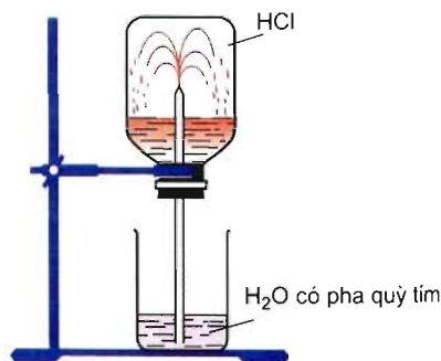
Hình 5.4. Thí nghiệm về tính tan của hiđro clorua
