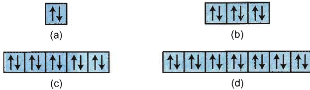
Hình 1.14. Số electron tối đa trong các phân lớp
