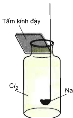
Hình 5.1. Natri cháy trong clo với ngọn lửa sáng
