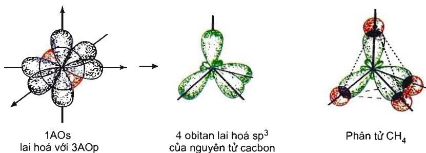
Hình 3.9. Sự lai hoá sp^3 và sự hình thành các liên kết trong phân tử CH_4 (góc liên kết H-C-H = 109^\circ 28' )
