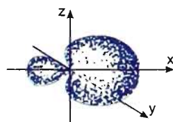
Hình 3.6. Dạng của một obitan lai hoá sp
