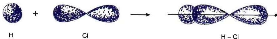
Hình 3.4. Sự xen phủ obitan 1s của hydro với obitan 3p của nguyên tử Cl tạo liên kết H – Cl
