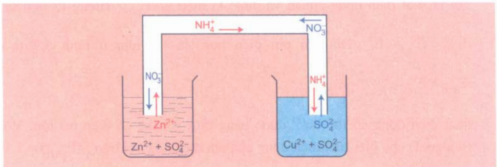
Hình 5.6. Sự di chuyển của các ion trong cầu muối khi pin hoạt động.
