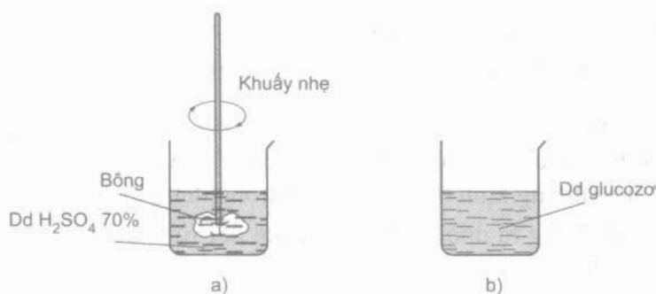
Hình 2.9. a) Thủy phân xenlulozơ
