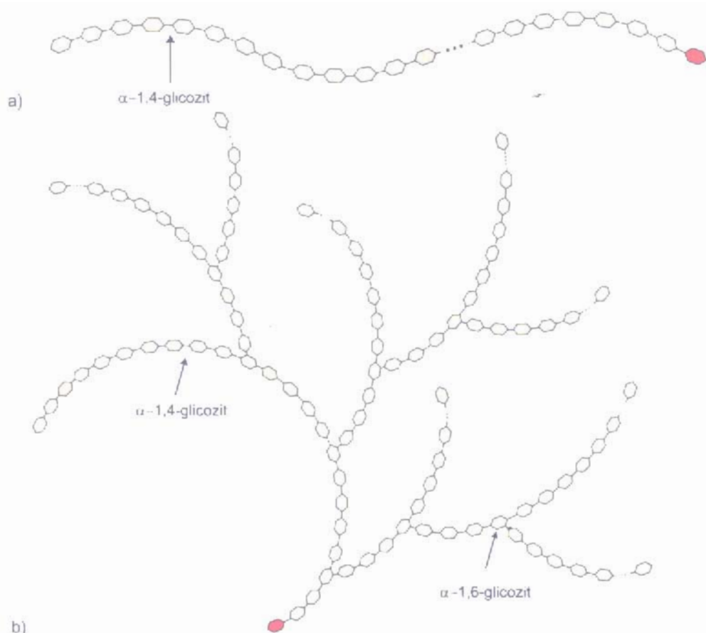
Hình 2.4. a) Mô hình phân tử amiloza ; b) Mô hình phân tử amilopectin
