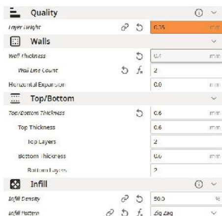
Hình 11.7. Giao diện cài đặt thông số in
