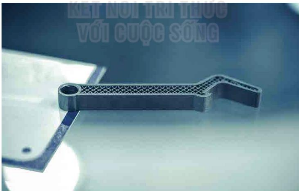
Hình 10.9. Sản phẩm in có kết cấu dạng lưới giảm trọng lượng
