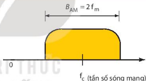
Hình 4.3. Băng thông của tín hiệu biên độ
