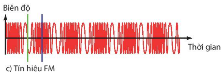
Hình 4.5. Biến điệu tần số
