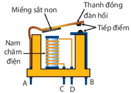
Hình 8.4. Cấu tạo của relay điện từ
