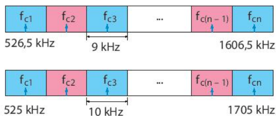
Hình 4.4. Cấp phát băng tần cho AM
