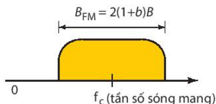
Hình 4.7. Băng thông của tín hiệu tần số
