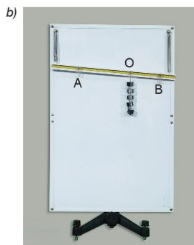
Hình 22.4. Thí nghiệm tổng hợp hai lực song song
