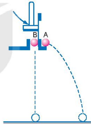
Hình 12.1. Thí nghiệm về chuyển động ném ngang
