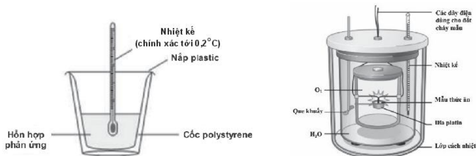
Hình 4.2. Cấu tạo của nhiệt lượng kế
