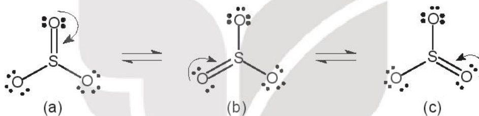
Hình 1.1. Cấu tạo cộng hưởng của phân tử \text{SO}_3
