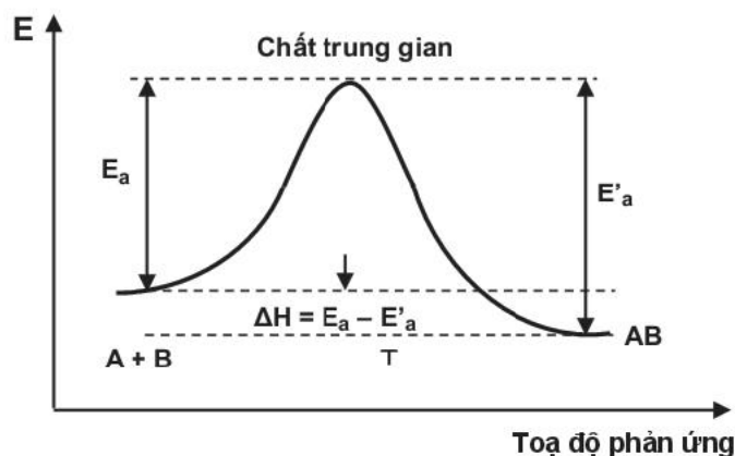
Hình 3.2. Giản đồ năng lượng của phản ứng (1)
