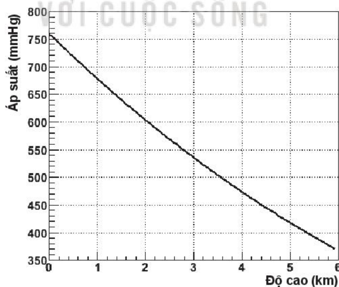
Hình 7.1. Sự phụ thuộc của áp suất vào độ cao
