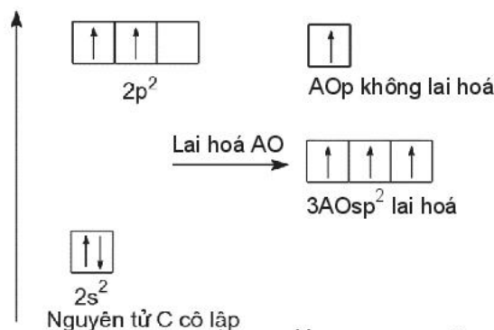
Hình 1.5. Giản đồ biểu diễn sự lai hoá AO của nguyên tử C tạo ra các AO lai hoá để tạo ra phân tử \text{C}_2\text{H}_4
