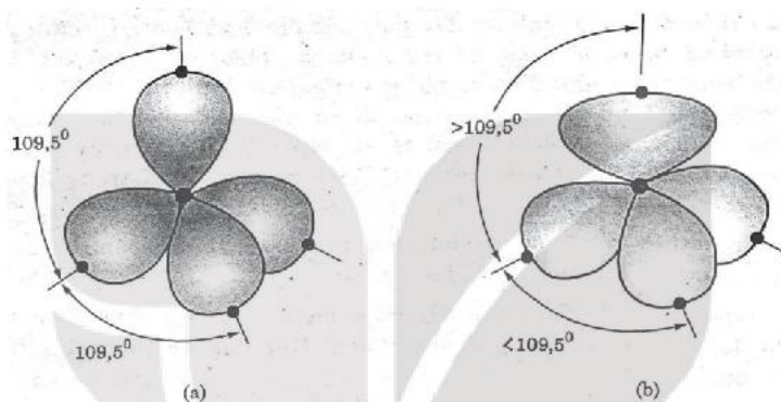
Hình 1.3. Vỏ electron hoá trị của nguyên tử trung tâm A
