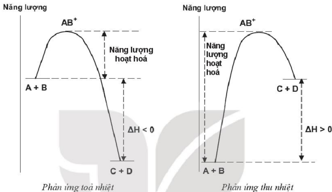
Hình 3.1. Đồ thị biểu diễn năng lượng hoạt hoá ( AB^+ là sản phẩm trung gian)
