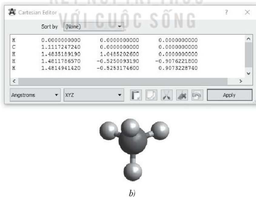
Hình 11.1. a) Cấu trúc hình học của phân tử \text{NH}_3 ; b) cấu trúc hình học phân tử \text{CH}_4
