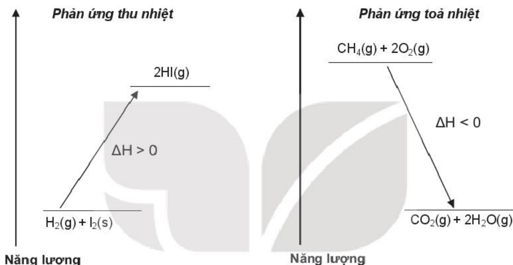
Bài 4.1. Sự biến thiên enthalpy đối với phản ứng thu nhiệt và phản ứng toả nhiệt
