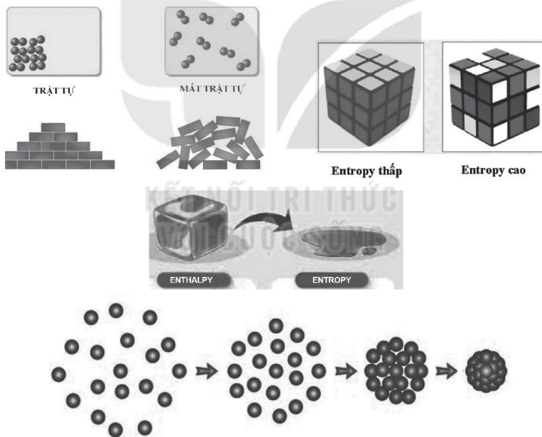
Hình 4.3. Một số hình ảnh về khái niệm entropy
