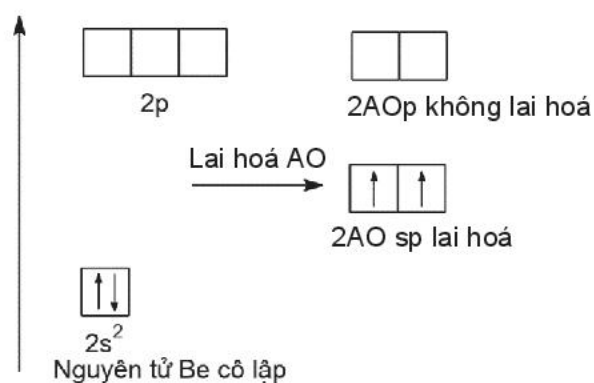
Hình 1.4. Giản đồ biểu diễn sự lai hoá AO của nguyên tử Be tạo ra các AO lai hoá để xen phủ với AO-s của nguyên tử H tạo ra phân tử BeH 2
