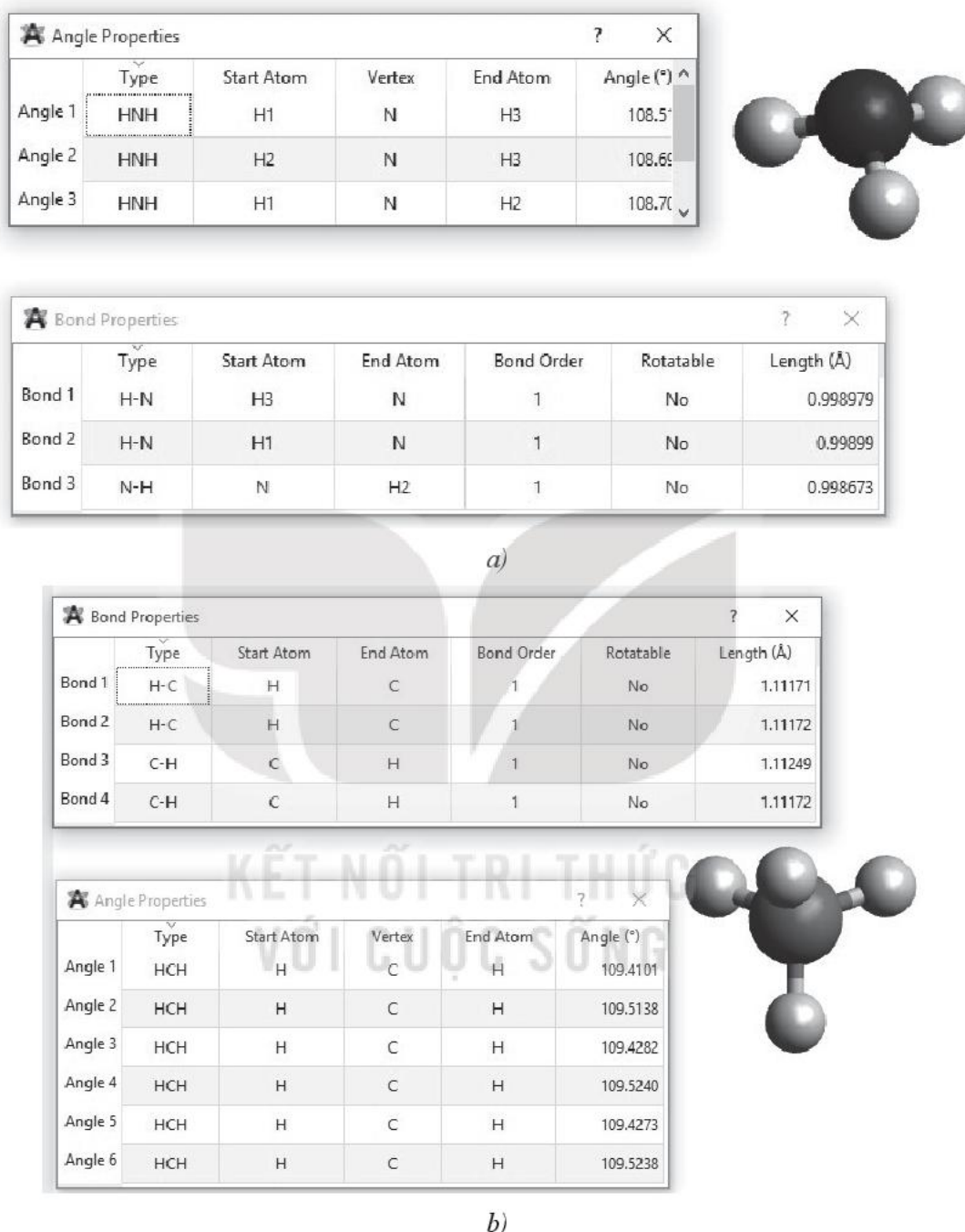
Hình 11.2. Hiển thị các tham số cấu trúc của a) phân tử \text{NH}_3 ; b) phân tử \text{CH}_4
