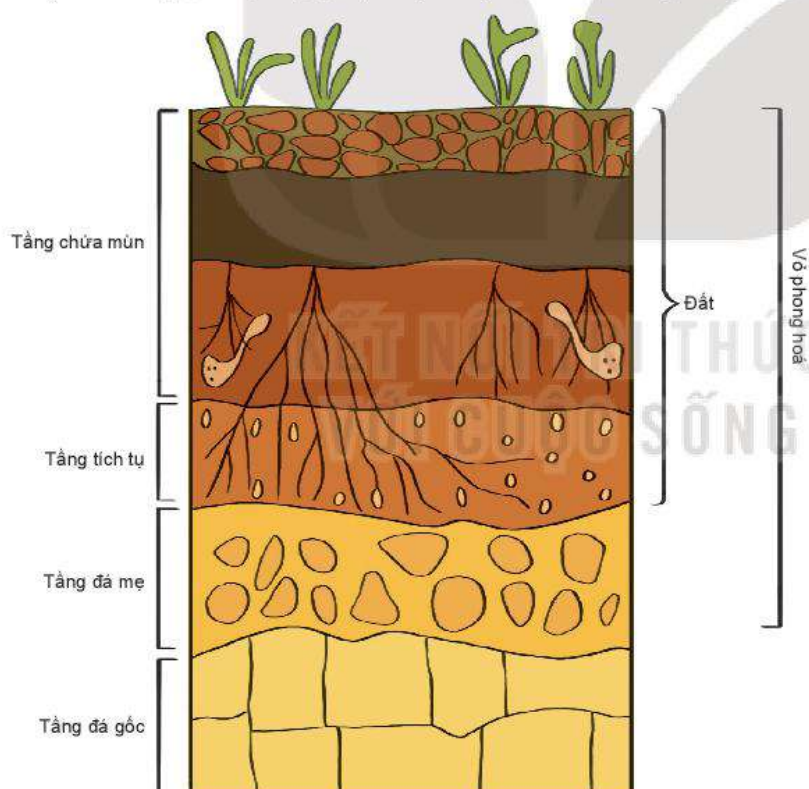
Hình 14.1. Phẫu diện đất và vỏ phong hoá
