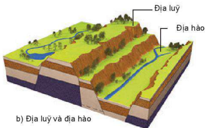
Hình 7.1. Hiện tượng uốn nếp và đứt gãy
