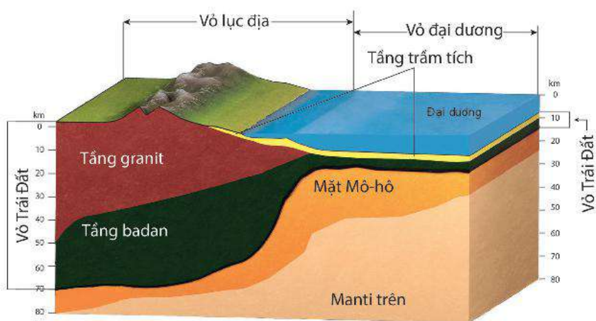
Hình 4. Sơ đồ cấu tạo vỏ Trái Đất
