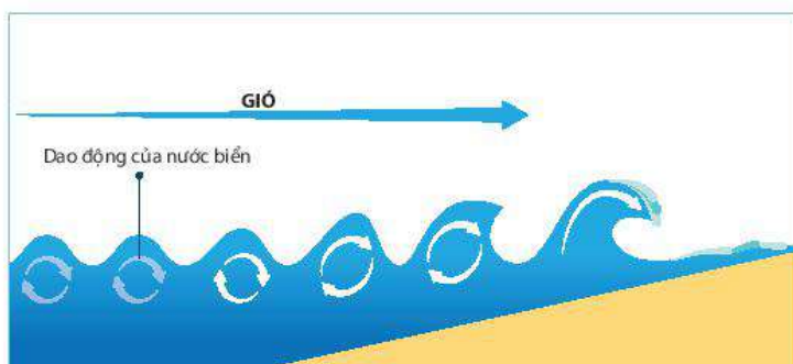
Hình 12.1. Sơ đồ sự hình thành sóng biển
