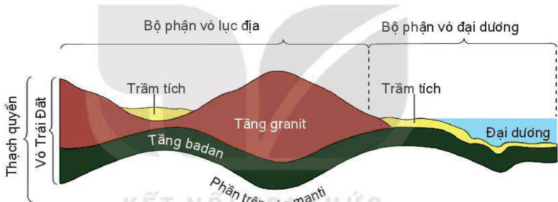
Hình 6.1. Vỏ Trái Đất và thạch quyển
