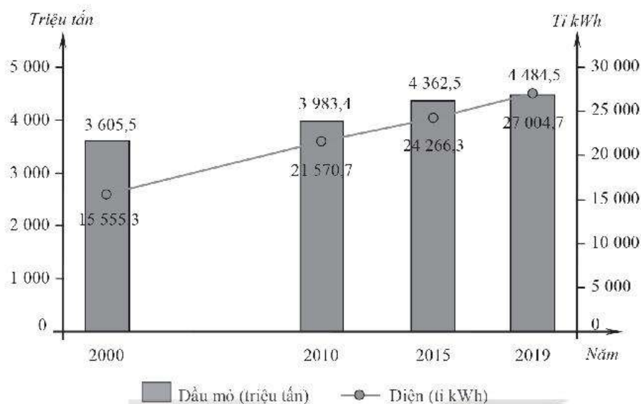
Biểu đồ sản lượng dầu mỏ và điện trên thế giới, giai đoạn 2000 – 2019
