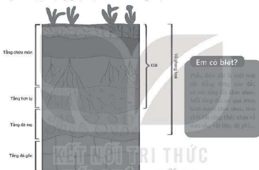
Hình 14.1. Phân diện đất và vỏ phong hoá
