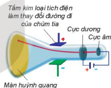
Hình 1.1. Thí nghiệm phát hiện hạt electron
