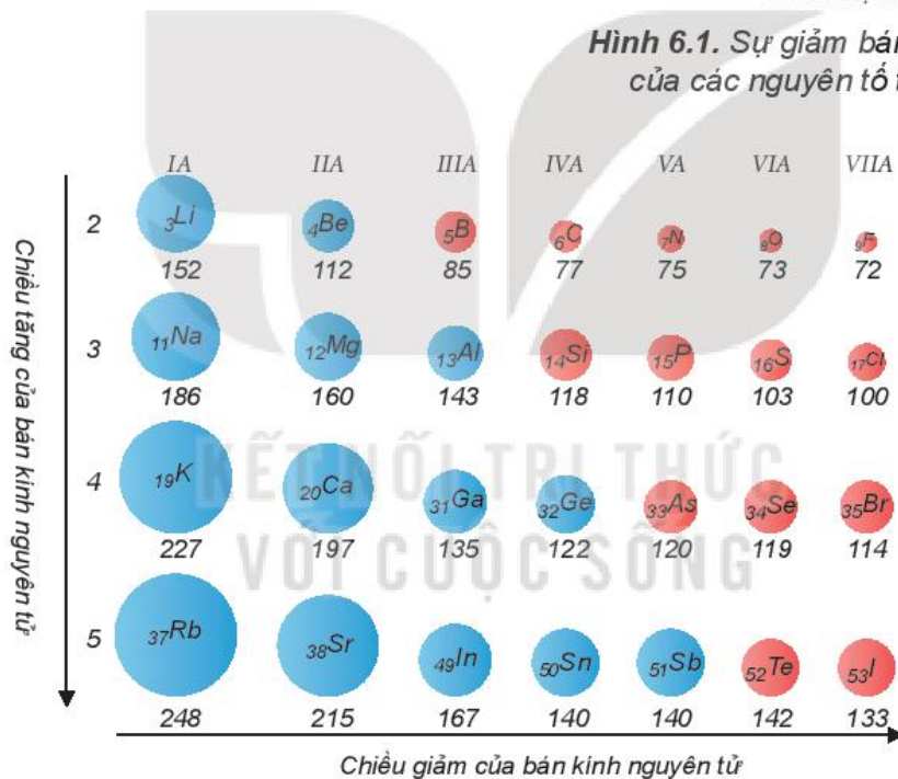
Hình 6.2. Giá trị bán kính nguyên tử (pm)(*)
