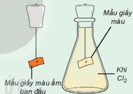
Hình 21.6. Tính tẩy màu của khí chlorine ẩm
