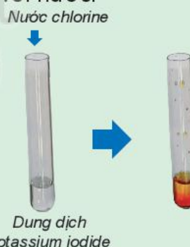
Hình 6.5. Phản ứng của nước chlorine với dung dịch potassium iodide
