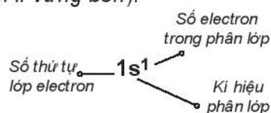
Hình 3.4. Cấu hình electron nguyên tử hydrogen
