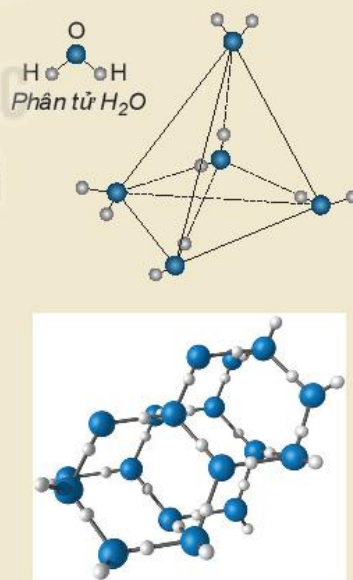
Hình 13.3. Mô hình cấu trúc nước đá
