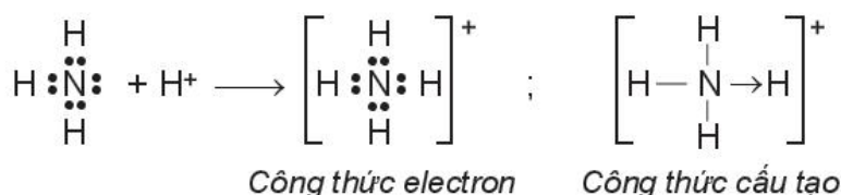
Hình 12.4. Sơ đồ sự tạo thành ion \text{NH}_4^+
