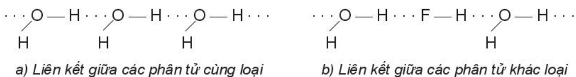
Hình 13.2. Hai kiểu tạo thành liên kết hydrogen
