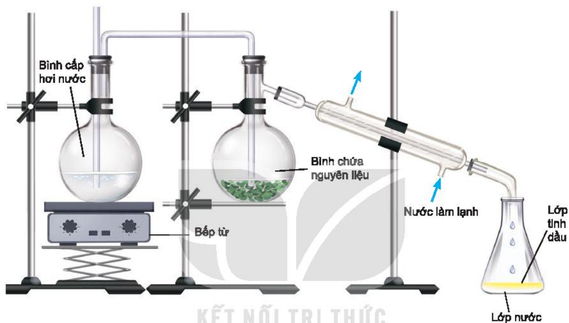
Hình 4.1. Thiết bị tách tinh dầu sả chanh bằng phương pháp chưng cất lôi cuốn hơi nước
