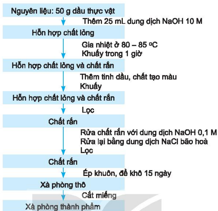
Hình 5.3. Sơ đồ chuyển hoá dầu thực vật thành xà phòng
