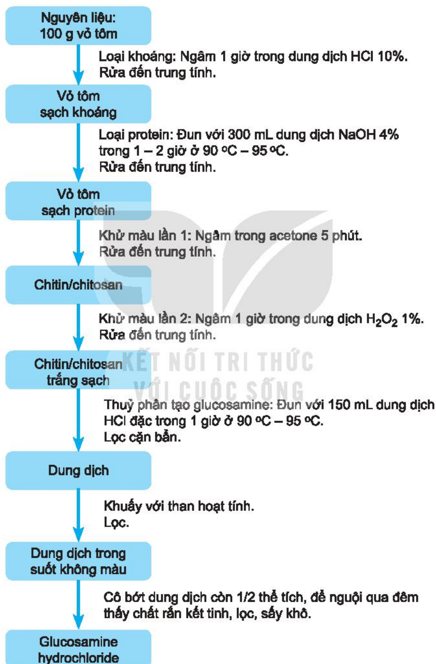
Hình 6.3. Sơ đồ điều chế glucosamine hydrochloride từ vỏ tôm
