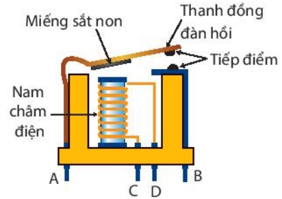
Hình 8.4. Cấu tạo của relay điện từ
