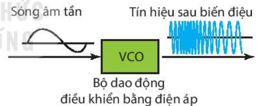
Hình 4.6. Sơ đồ nguyên lí biến điệu tần số
