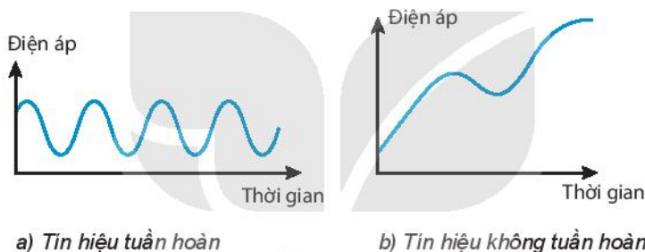
Hình 5.1. Tín hiệu tương tự
