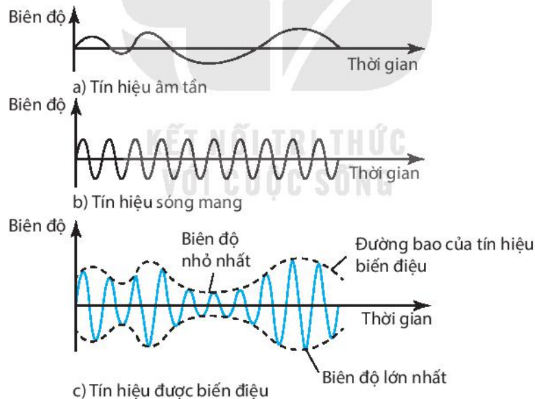
Hình 4.1. Biến điệu biên độ
