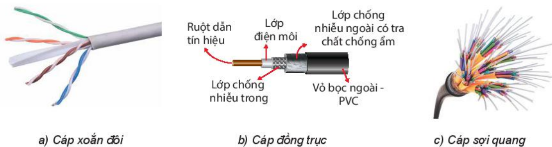
Hình 6.3. Các loại cáp truyền dẫn
