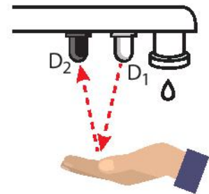
Hình 9.9. Mô hình vòi nước rửa tay tự động: D_1 là diode phát hồng ngoại, D_2 là diode thu hồng ngoại
