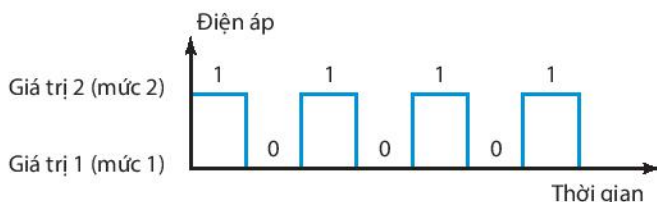
Hình 5.2. Tín hiệu số
