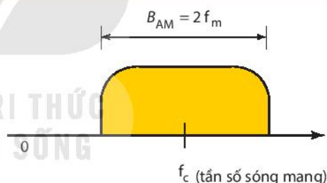
Hình 4.3. Băng thông của tín hiệu AM
