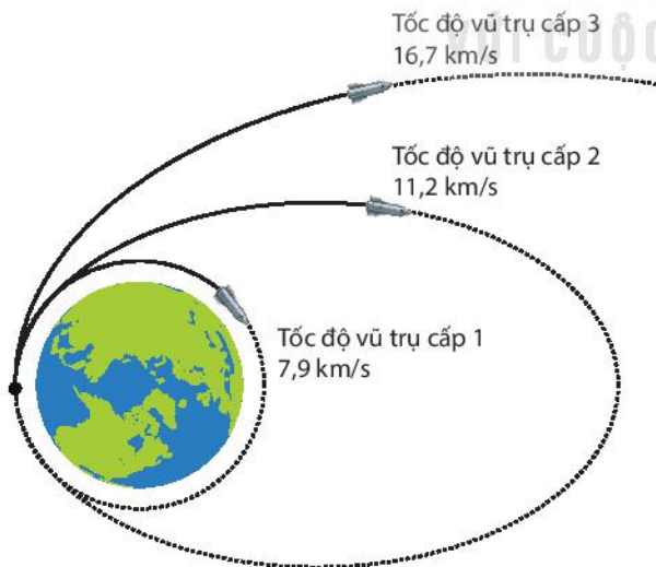
Hình 3.8. Minh hoạ mô phỏng quỹ đạo của vật được phóng với tốc độ khác nhau từ Trái Đất
