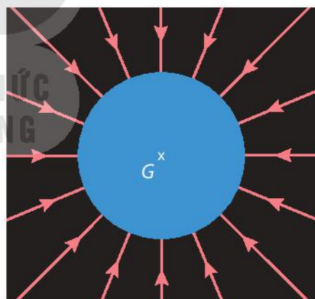
Hình 2.2. Biểu diễn đường sức trường hấp dẫn
