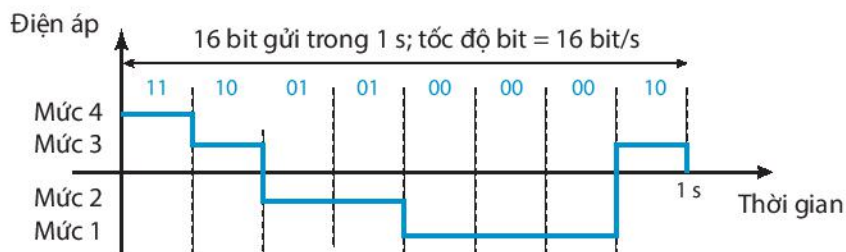
b) Tín hiệu số với bốn mức
