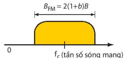
Hình 4.7. Băng thông của tín hiệu FM
