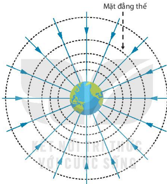
Hình 3.3. Mặt đẳng thế
