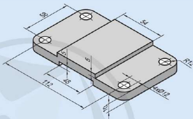
Hình 14.6. Tấm đế
