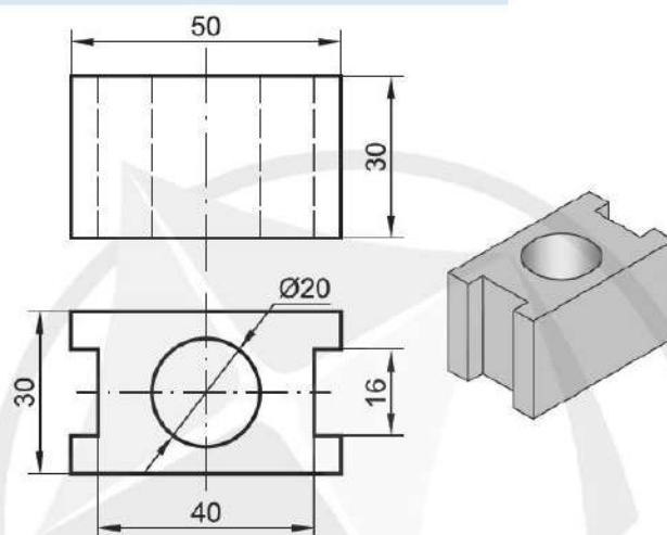
Hình 10.10. Con trượt
