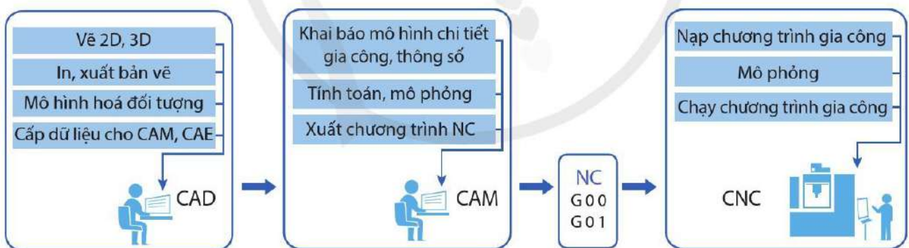
Hình 6.2. Sơ đồ hệ thống CAD/CAM–CNC
