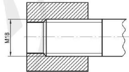
Hình 13.5. Vẽ quy ước mối ghép ren
