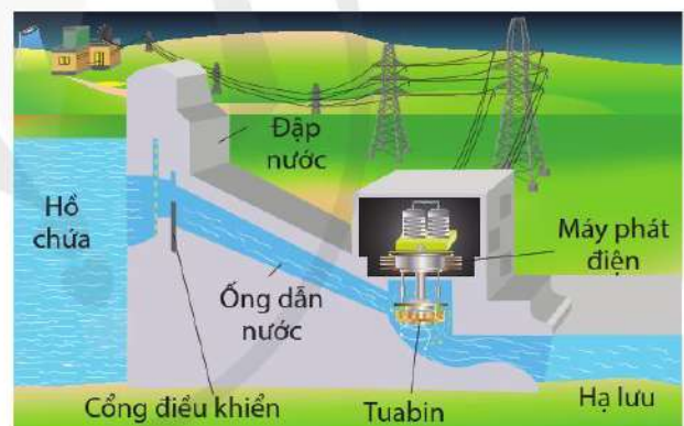
Hình 3.11. Sơ đồ nhà máy thủy điện
