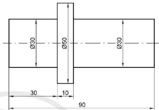
Hình 11.6. Trục
