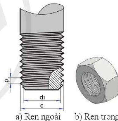
Hình 13.2. Ren ngoài và ren trong
