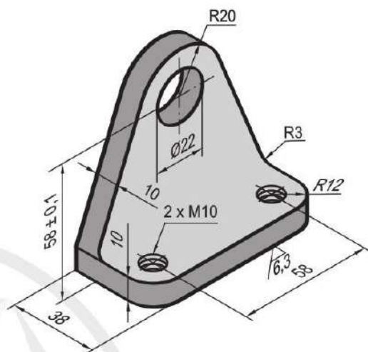
Hình 14.1. Càng đỡ
