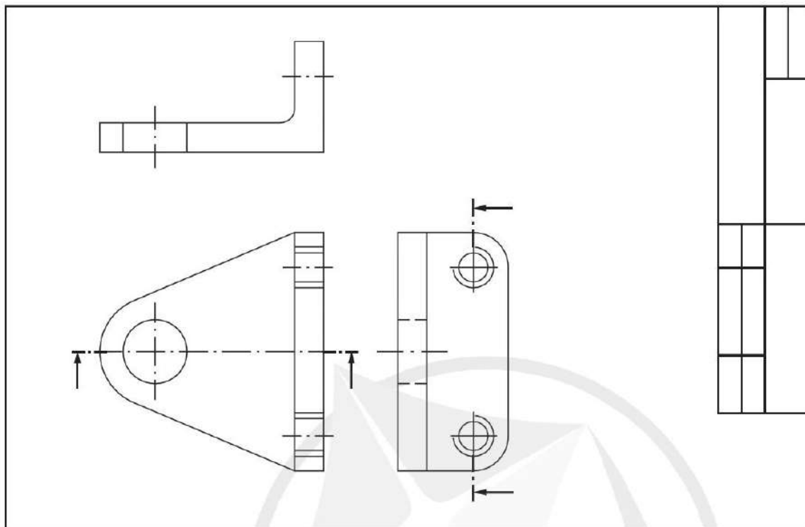
Hình 14.3. Vẽ mờ
