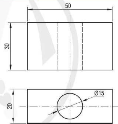
Hình 17.8. Gõ cột
