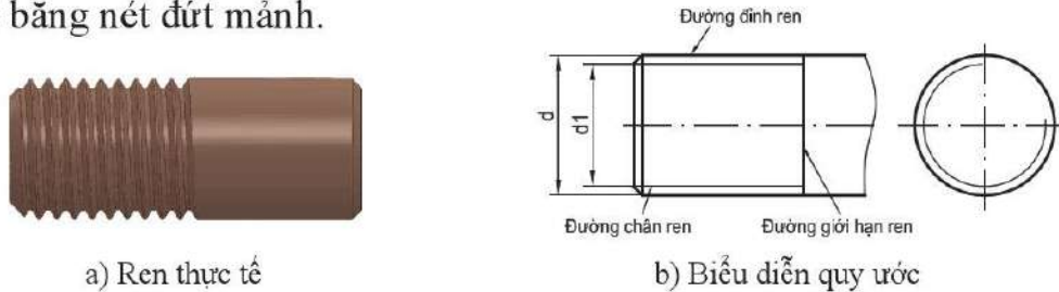
Hình 13.3. Biểu diễn ren trục
