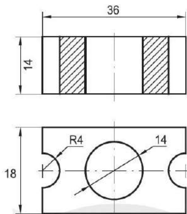
Hình 03.1. Ghi kích thước cho bản vẽ
