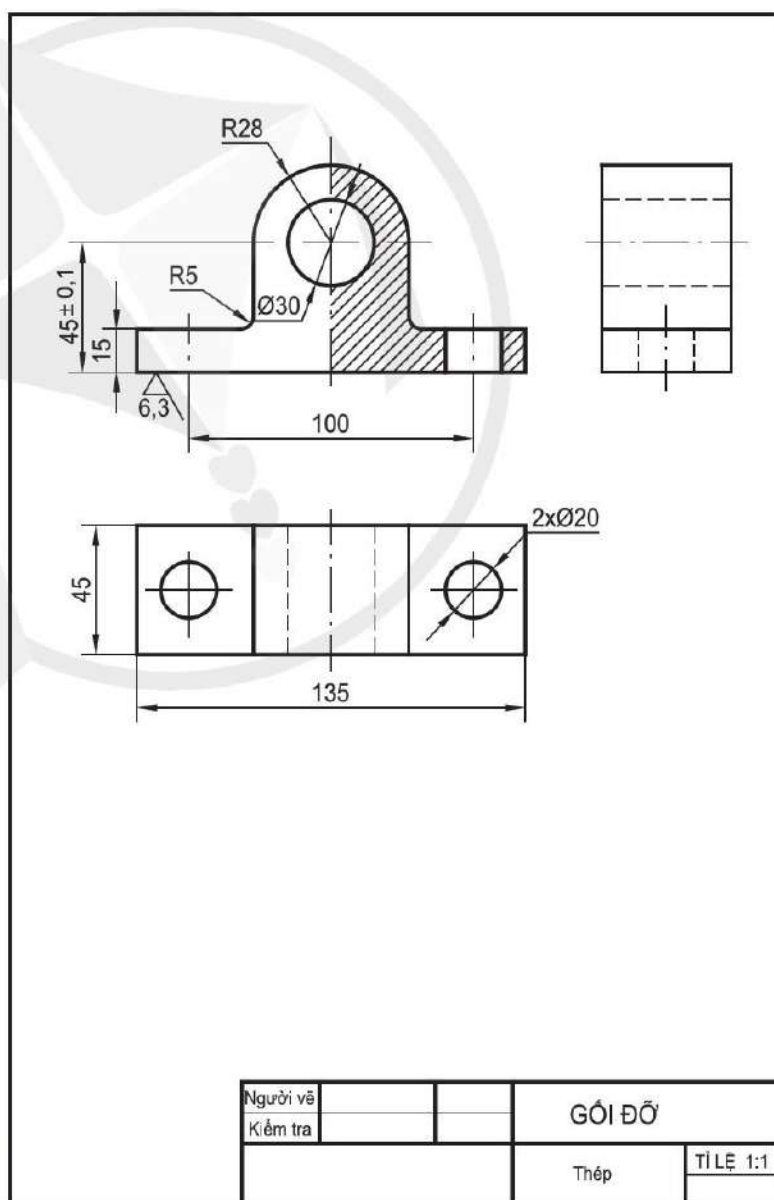
Hình 19.1. Bản vẽ gôi đỡ
