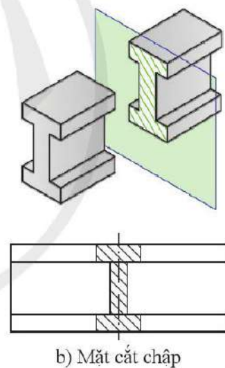
Hình 10.4. Các loại mặt cắt
