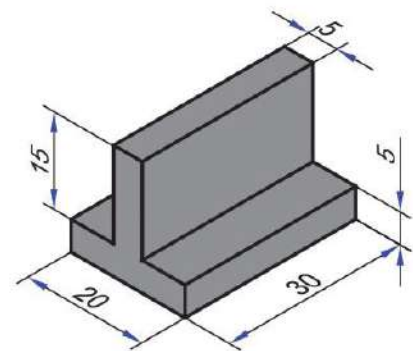
Hình 10.5. Khối thép hình chữ T
