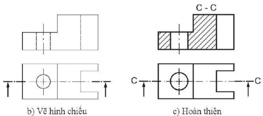
Hình 10.9. Vẽ hình cắt
