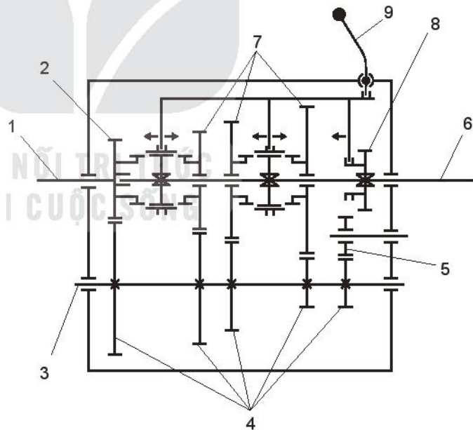
Hình 22.4. Hộp số thường ba trục
