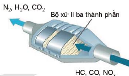
Hình 20.12. Cấu tạo của bộ xử lí ba thành phần
