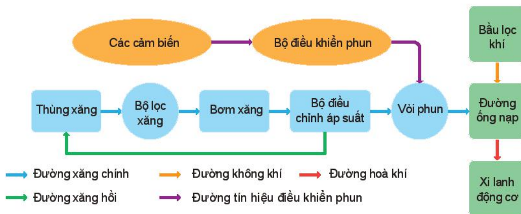
Hình 20.6. Sơ đồ hệ thống phun xăng
