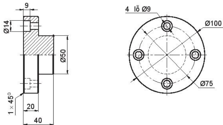
Hình 9.2. Hình vẽ chi tiết mặt bích
