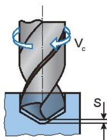
Hình 8.5. Thông số chế độ cắt khi khoan
