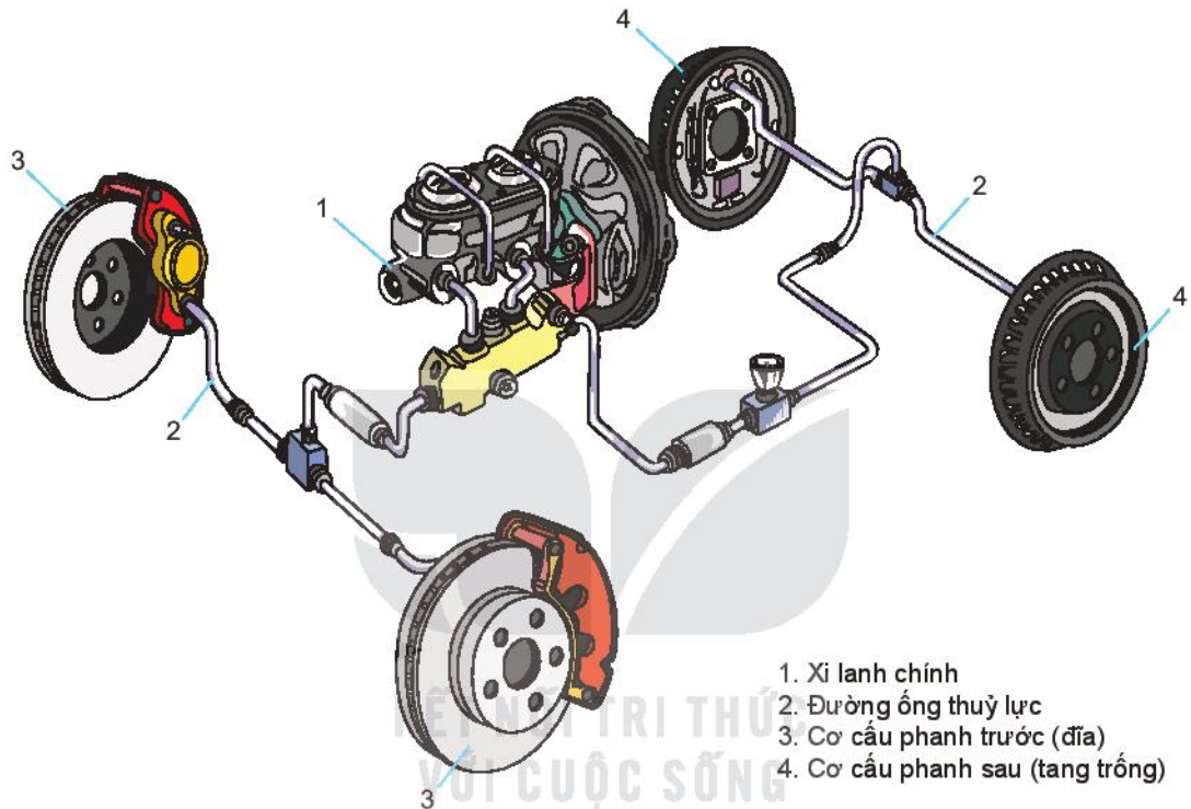
Hình 25.2. Hệ thống phanh trên ô tô con
