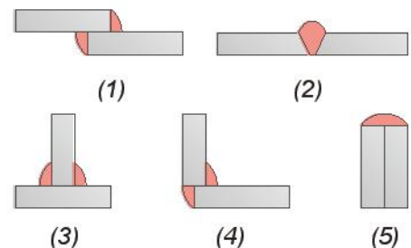
Hình 8.4. Các kiểu liên kết hàn
