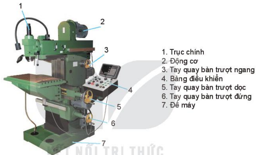
Hình 8.9. Máy phay đứng vạn năng
