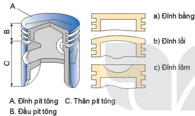
Hình 19.3. Cấu tạo pít tông
