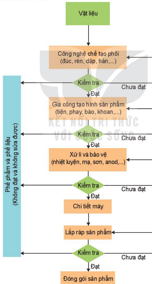
Hình 11.2. Quá trình sản xuất cơ khí
