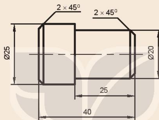
Hình 9.11. Hình vẽ chi tiết chốt
