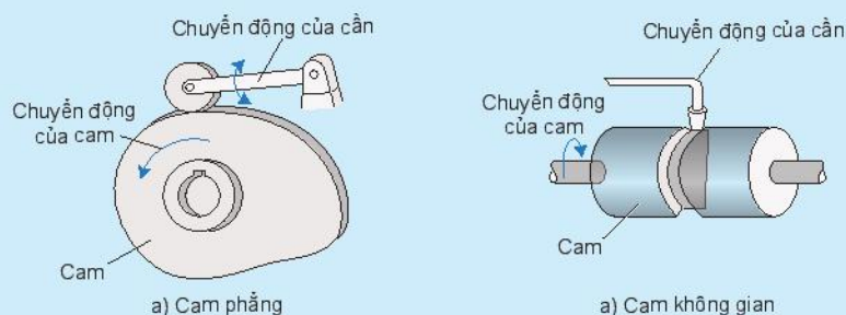
Hình 12.4. Một số nguyên lý cơ cấu cam
