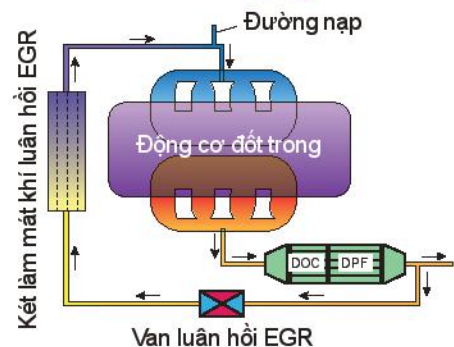
Hình 20.11. Hệ thống luân hồi EGR kết hợp bộ DOC và DPF
