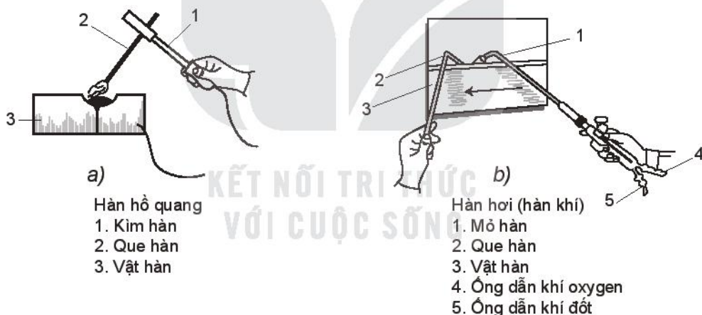
Hình 8.3. Một số phương pháp hàn thông dụng
