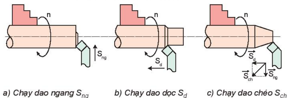
Hình 8.8. Các chuyển động khi tiện
