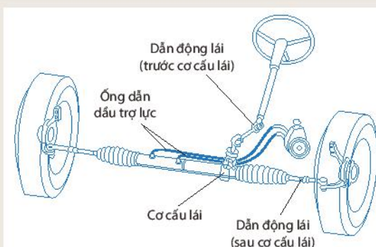
Hình 24.2. Cấu tạo chung của hệ thống lái
