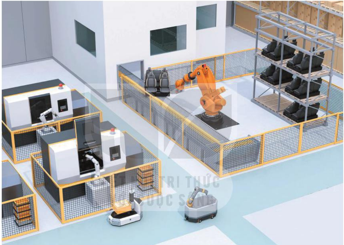
Hình 12.7. Một phần dây chuyền sản xuất tự động mềm
