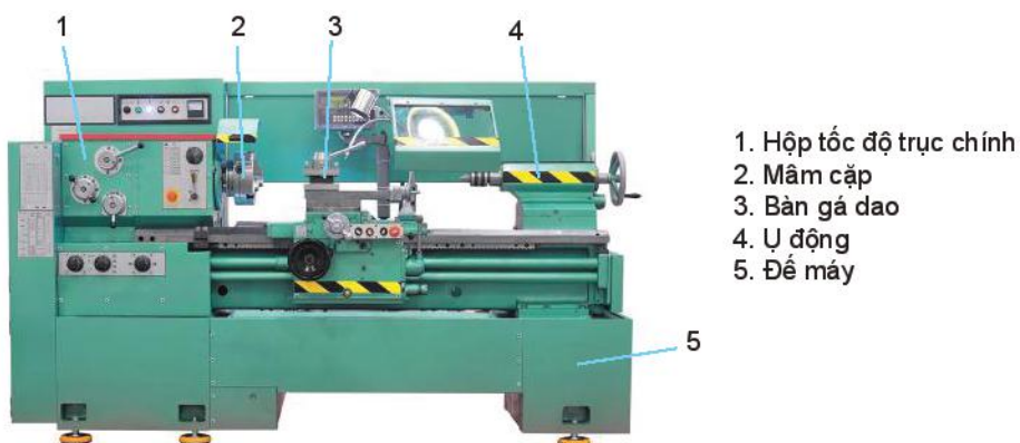
Hình 8.7. Máy tiện vạn năng
