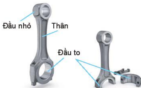
Hình 19.4. Cấu tạo thanh truyền
