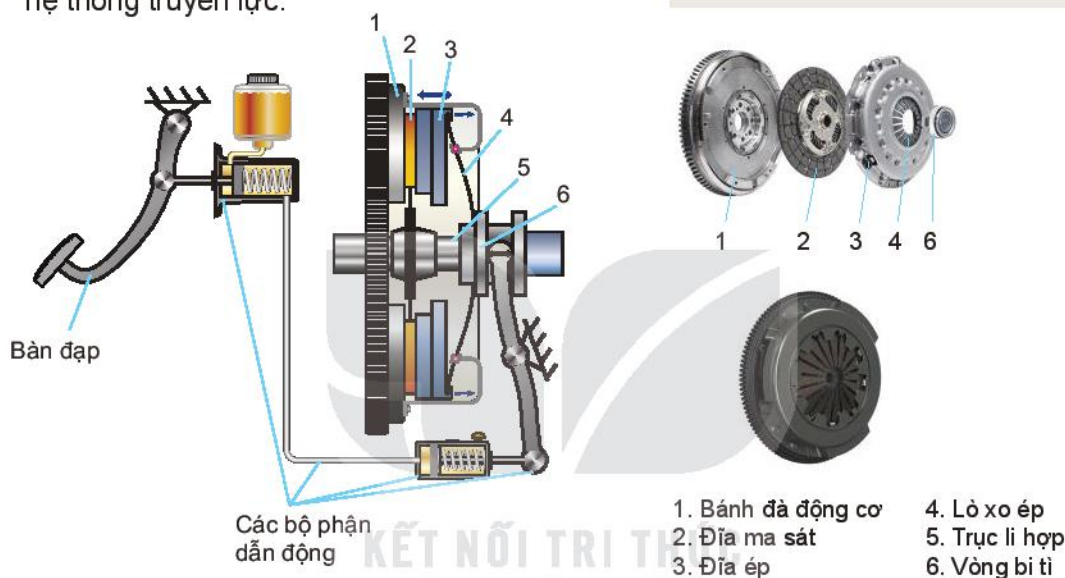
Hình 22.3. Li hợp ô tô con
