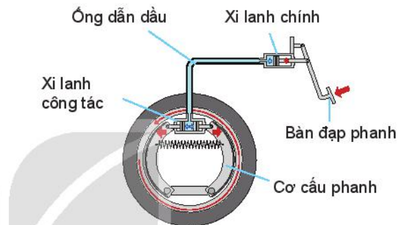
Hình 21.6. Hệ thống phanh
