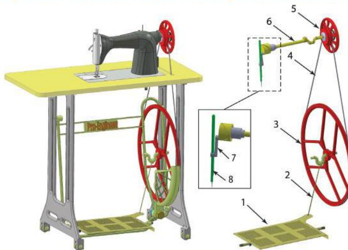
Hình 6.8. Máy may đạp chân:
