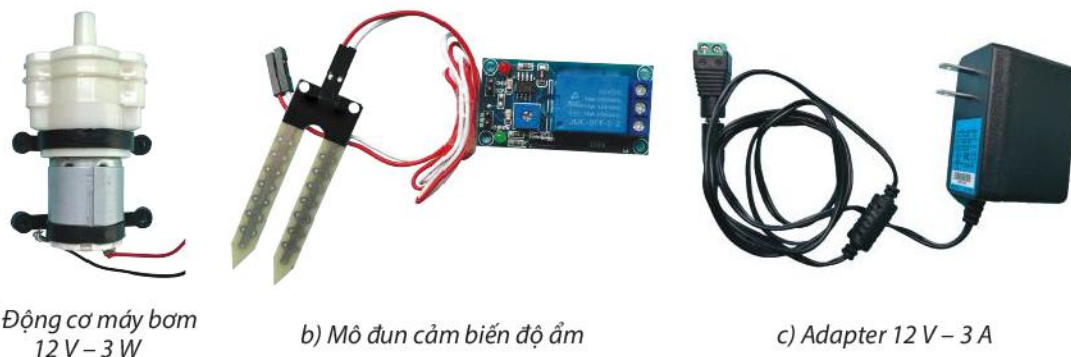
Hình 11.6. Thiết bị, vật liệu chính để lắp ráp mạch điện điều khiển sử dụng mô đun cảm biến độ ẩm
