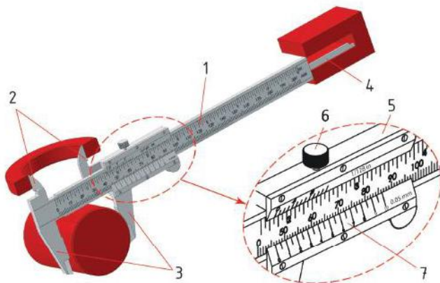
Hình 5.3. Thước cặp
