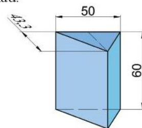
Hình 2.11. Hình lăng trụ tam giác đều
