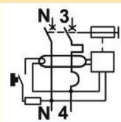
Hình 8.4. Kí hiệu Aptomat chống giật
