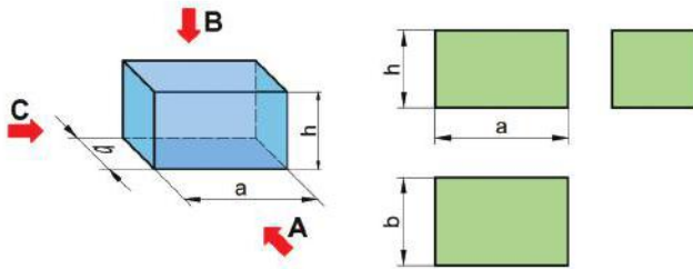
Hình 2.8. Hình chiếu của hình hộp chữ nhật
