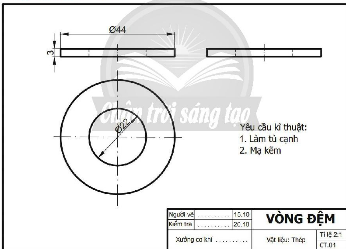
Hình 3.2. Bản vẽ chi tiết vòng đệm
