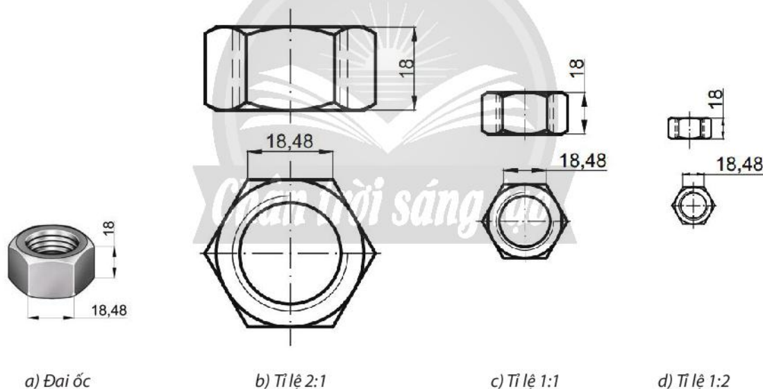
Hình 1.3. Đai ốc và tỷ lệ hình biểu diễn của đai ốc trên bản vẽ
