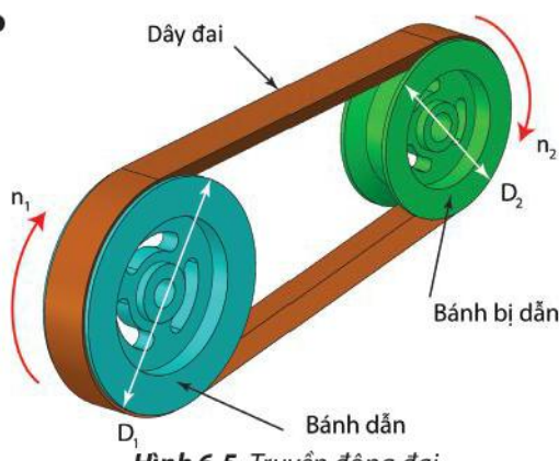
Hình 6.5. Truyền động đai
