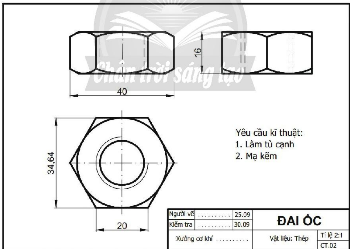
Hình 3.5. Bản vẽ chi tiết đai ốc
