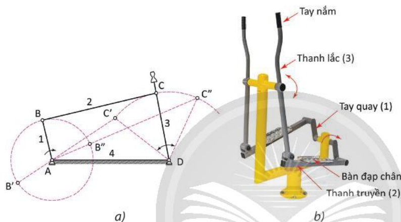
Hình 6.7. Cơ cấu tay quay thanh lắc (a)
