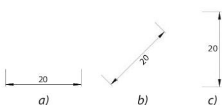
Hình 1.5. Ghi chữ số kích thước
