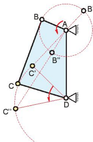
a) Cơ cấu tay quay thanh lắc
