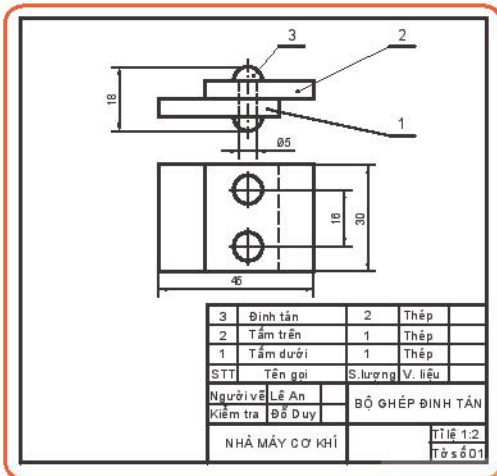
Hình 4.1. Nội dung của bản vẽ bộ định tán
