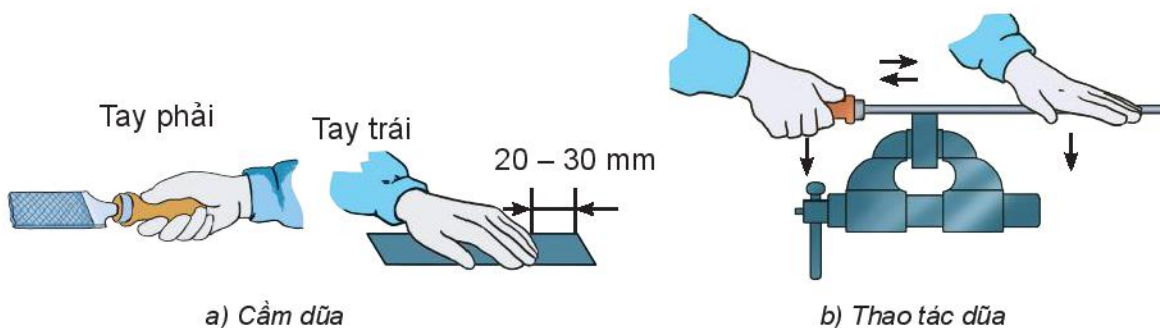
Hình 8.12. Cầm dũa và thao tác dũa
