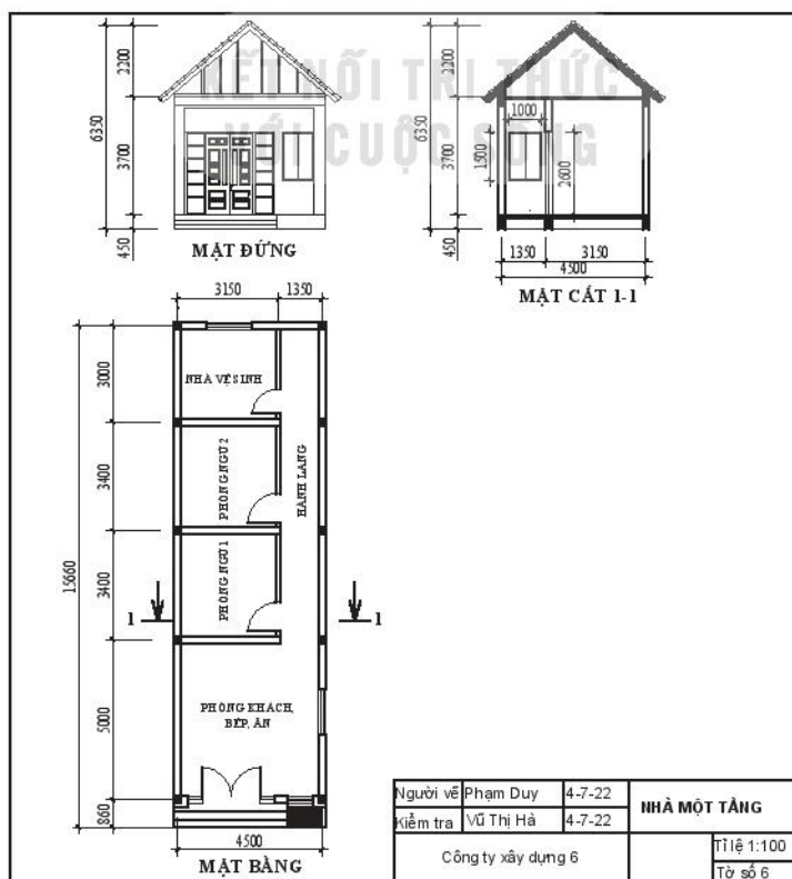
Hình 5.3. Bản vẽ nhà một tầng
