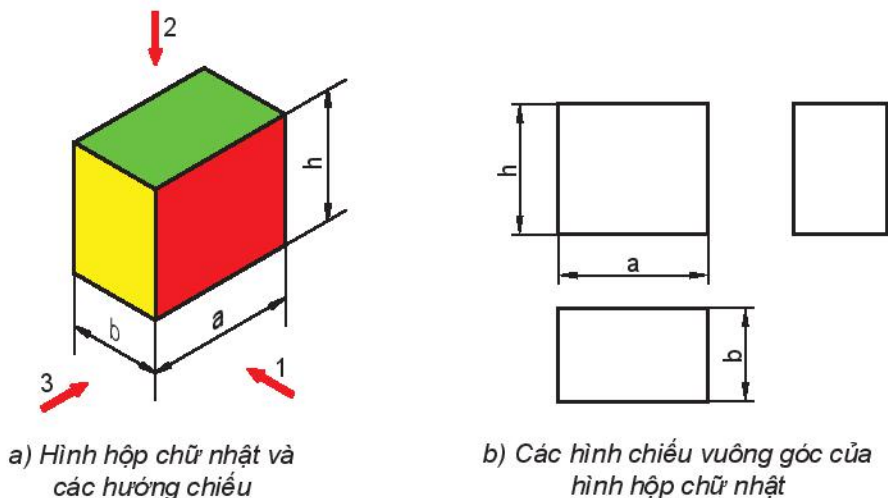
Hình 2.7. Hình hộp chữ nhật và các hình chiếu vuông góc
