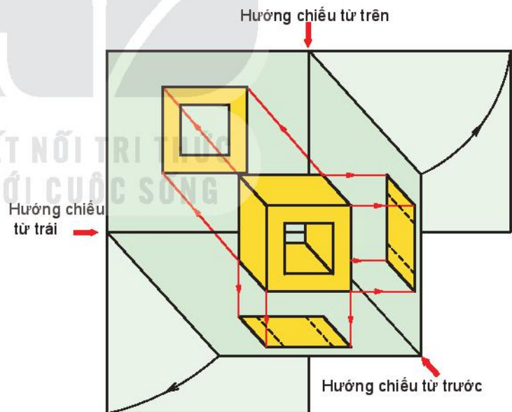
Hình 2.4. Các hình chiếu và hướng chiếu
