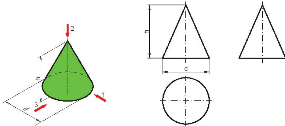
a) Hình nón và các hướng chiếu
