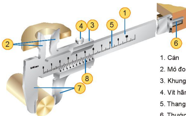
Hình 8.4. Cấu tạo của thước cặp
