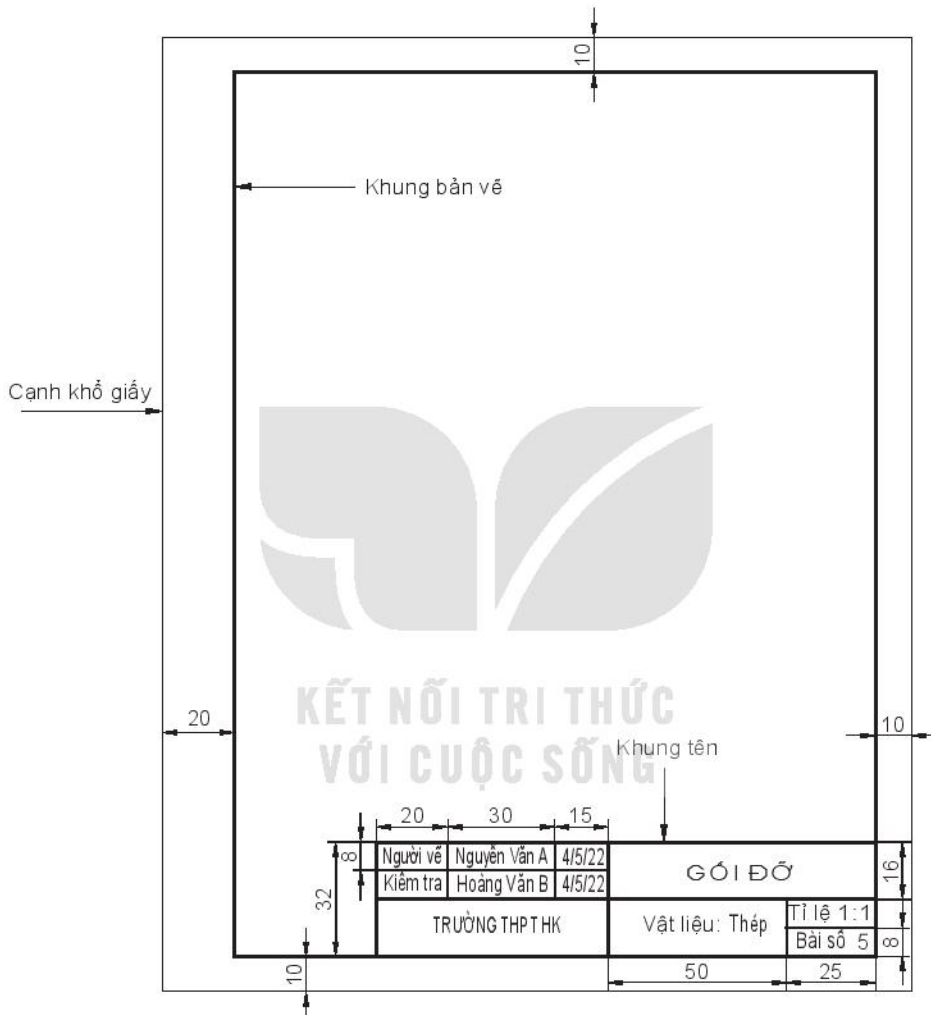
Hình 1.3. Khung bản vẽ, khung tên
