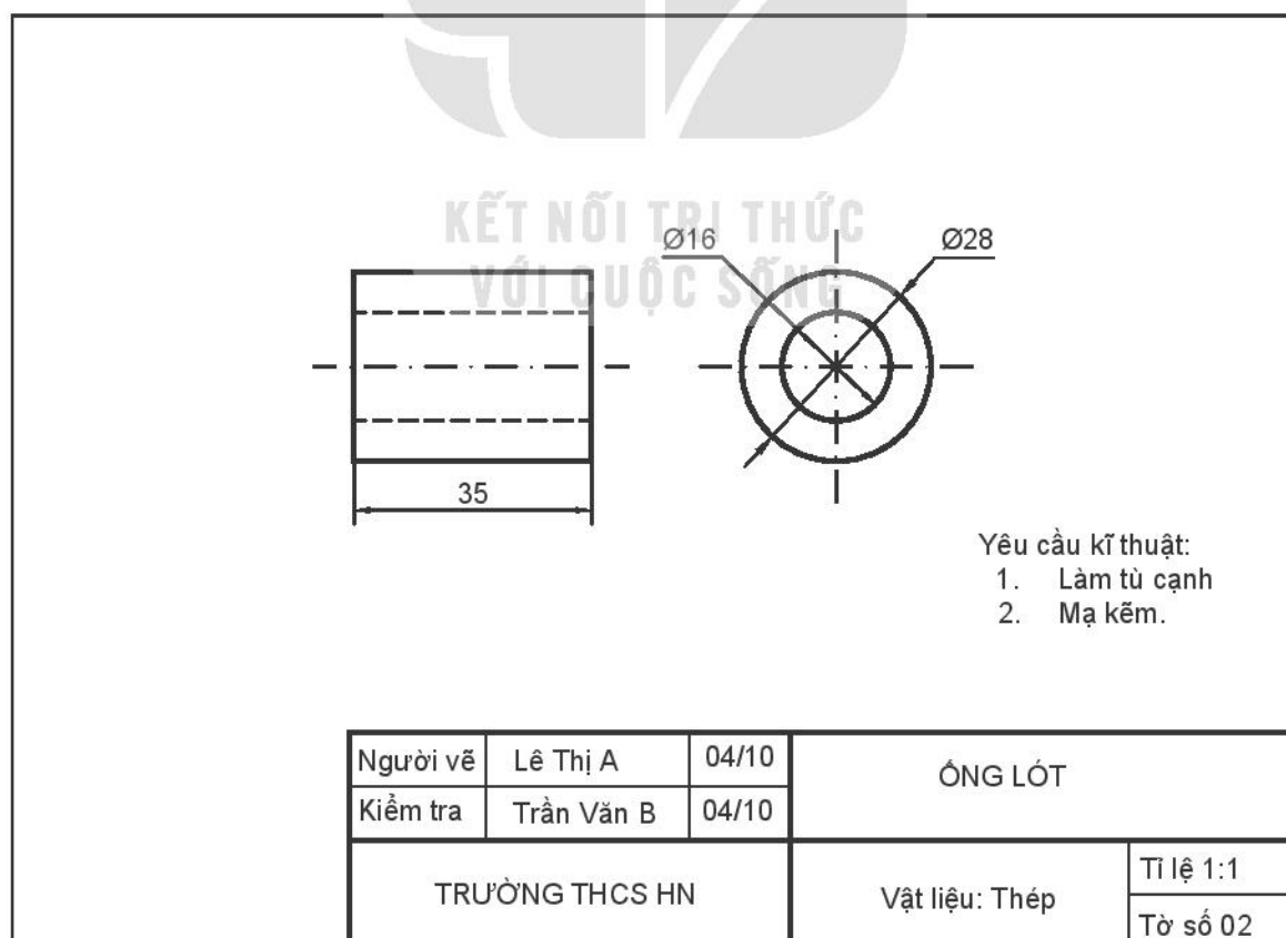
Hình 3.5. Bản vẽ ống lót
