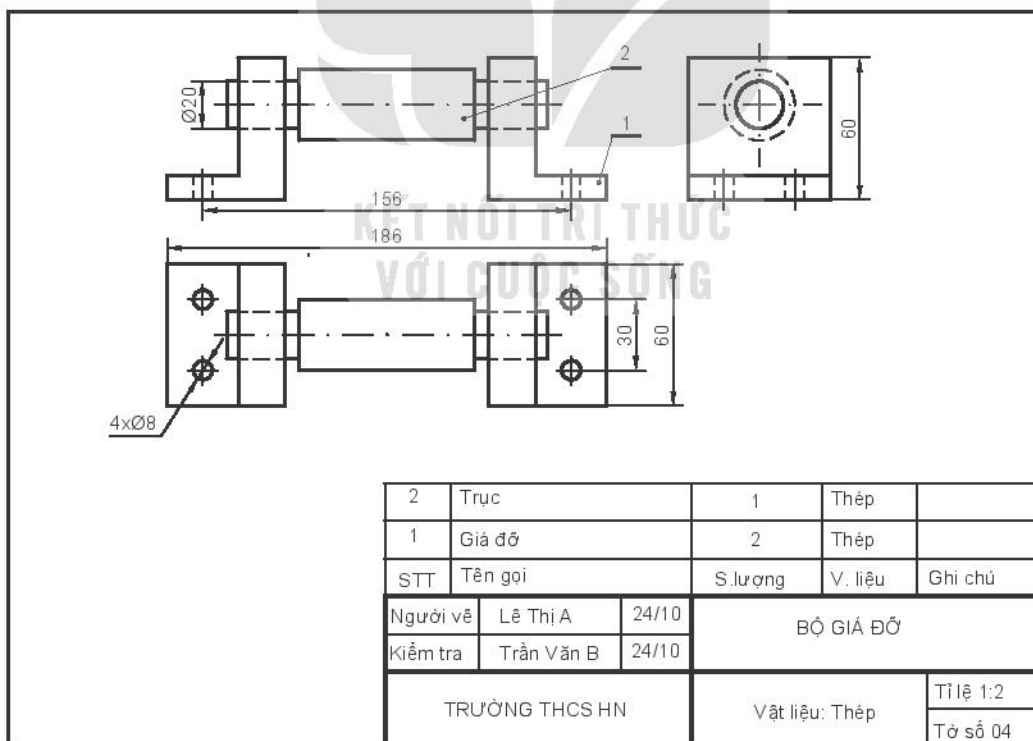
Hình 4.8. Bản vẽ lắp bộ giá đỡ
