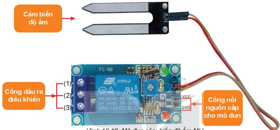
Hình 16.10. Mô đun cảm biến độ ẩm MH
