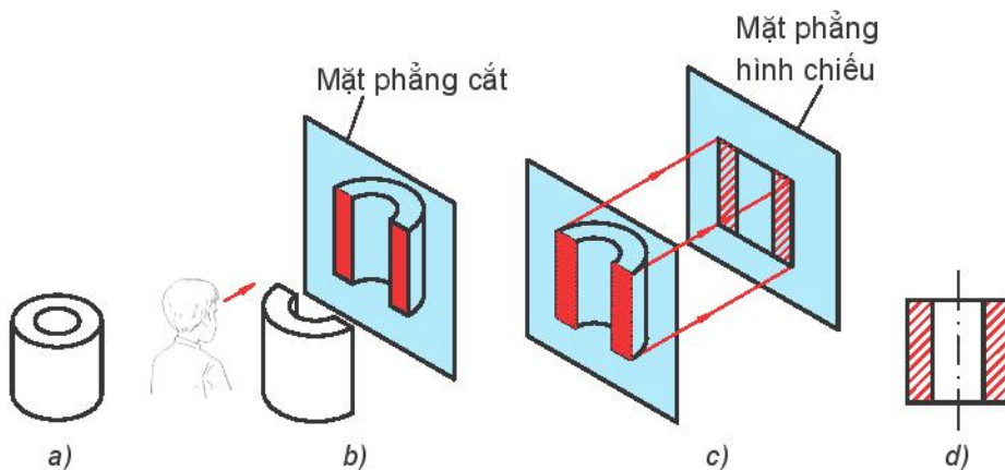
Hình 3.4. Phương pháp hình cắt
