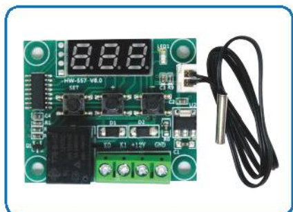
Hình 16.1. Mô đun cảm biến nhiệt độ
