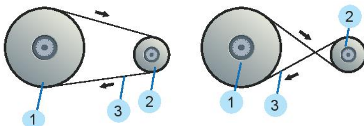
a) Truyền động dây đai thẳng
