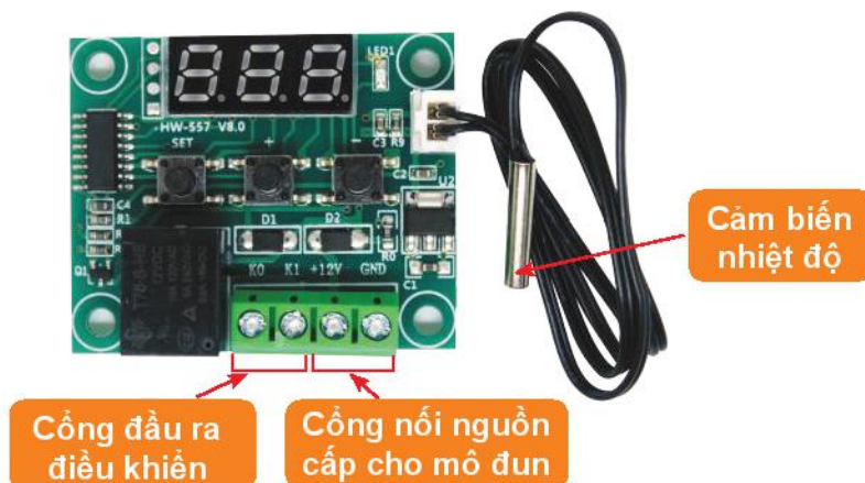
Hình 16.7. Mô đun cảm biến nhiệt độ XH W1209
