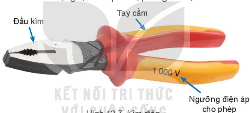
Hình 12.7. Kim điện
