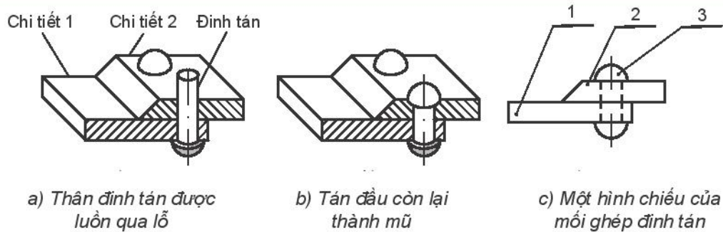
Hình 4.3. Mối ghép đinh tán
