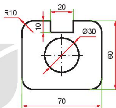
Hình 1.5. Ghi kích thước
