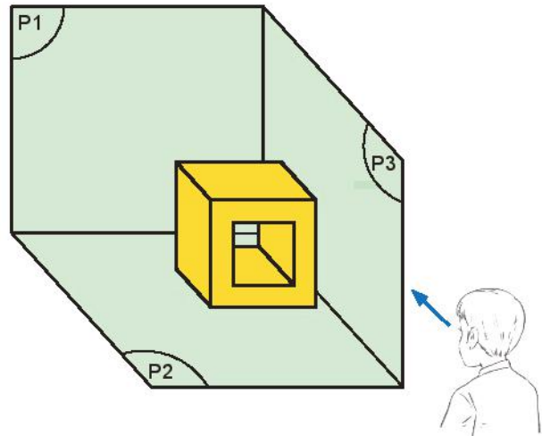
Hình 2.3. Các mặt phẳng hình chiếu
