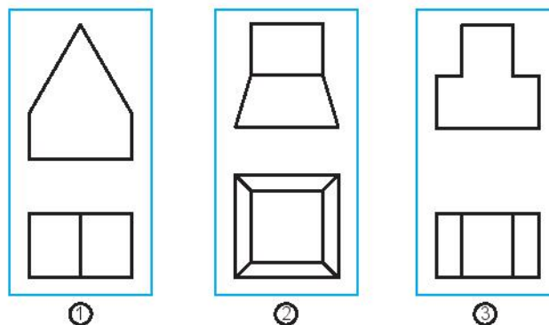
Hình 2.11. Các cặp hình chiếu
