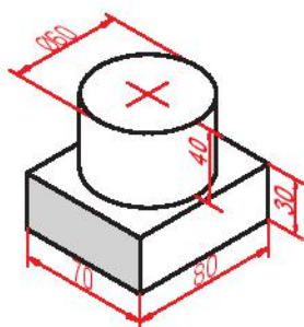
Hình 2.19. Gối đỡ
