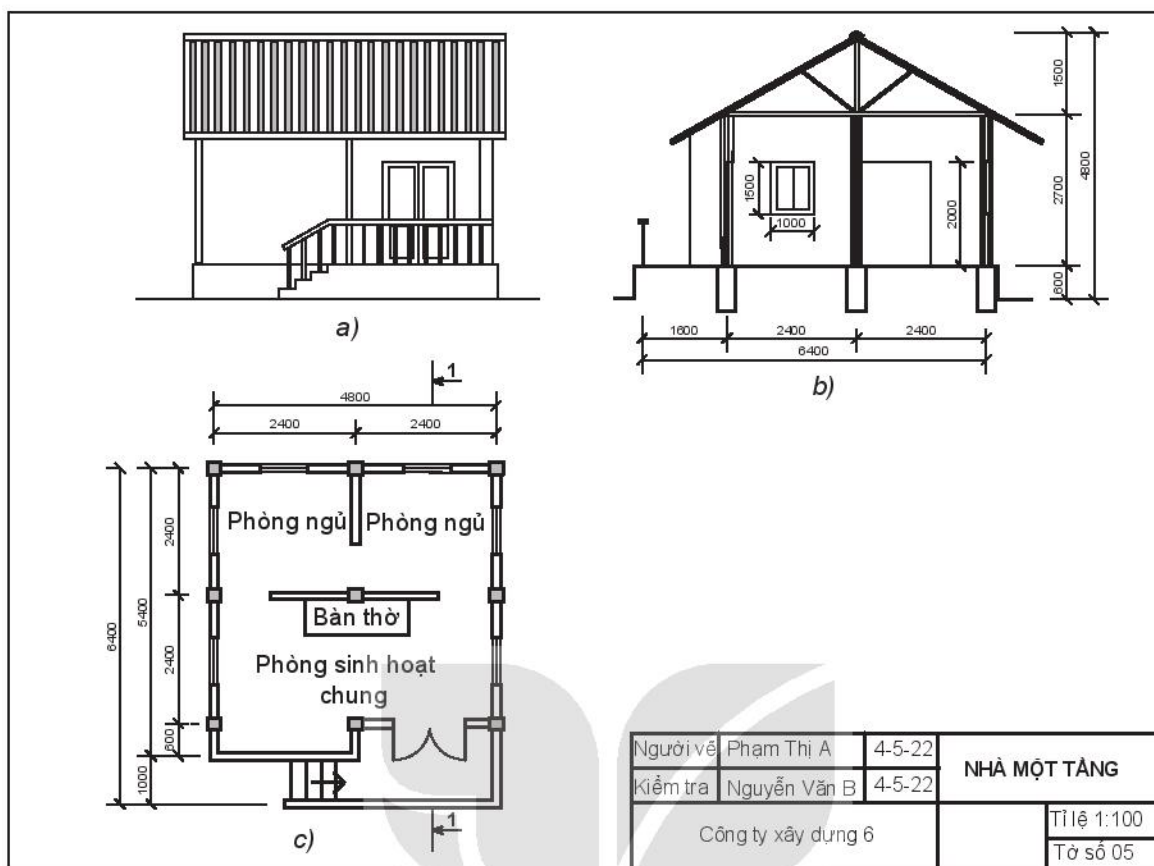
Hình 5.2. Một số hình biểu diễn của ngôi nhà
