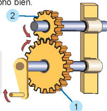
1. Bánh dẫn; 2. Bánh bị dẫn
