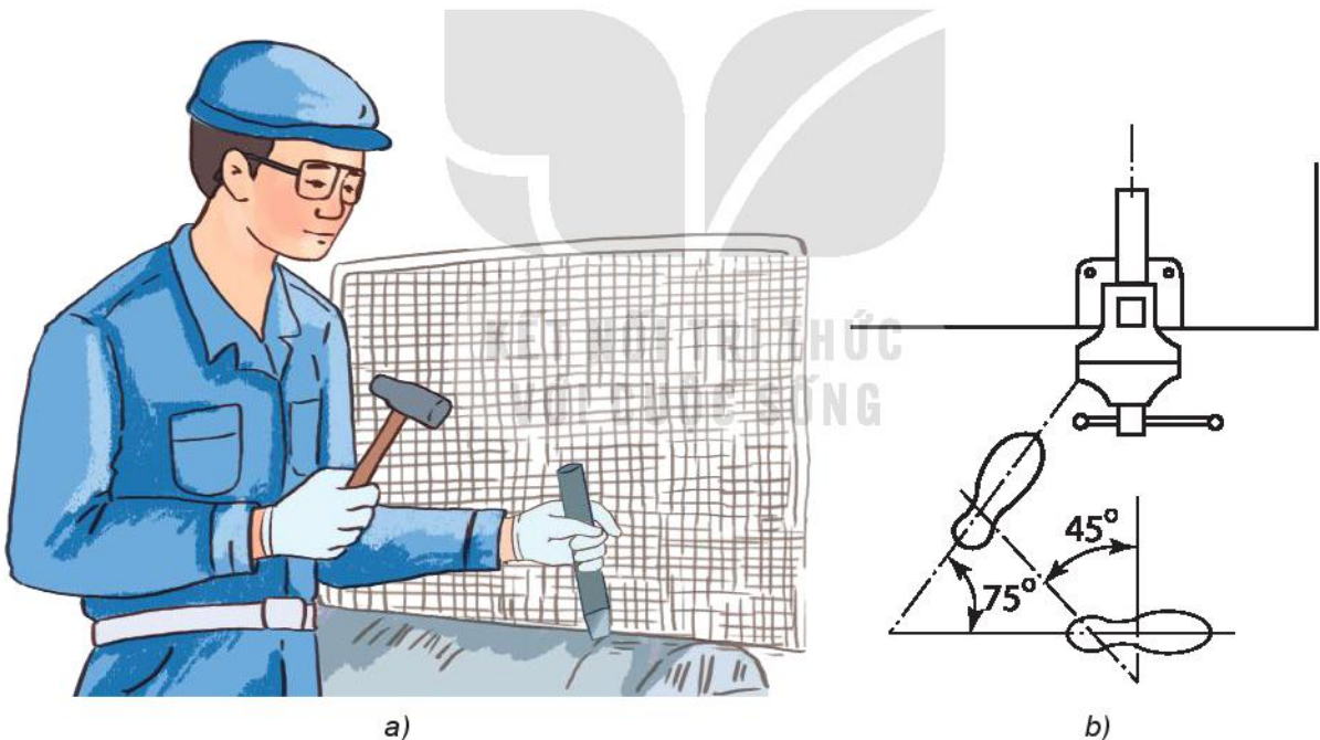
Hình 8.10. Tư thế đục và vị trí chân
