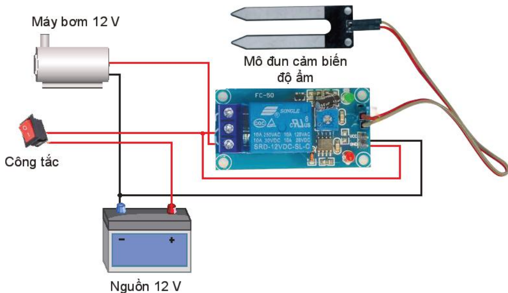
Hình 16.11. Sơ đồ lắp ráp mạch điện điều khiển máy bơm sử dụng mô đun cảm biến độ ẩm
