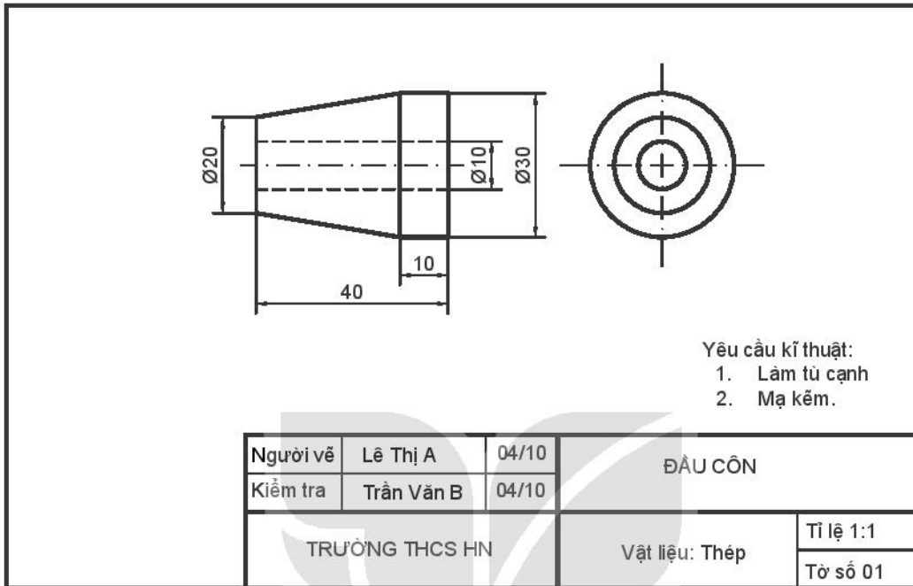
Hình 3.3. Bản vẽ đầu côn
