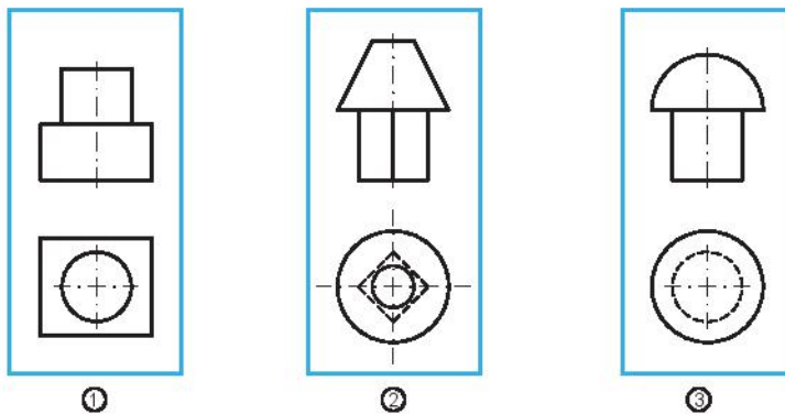
Hình 2.18. Các cặp hình chiếu
