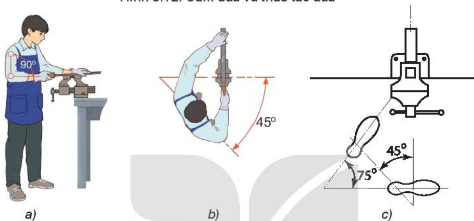
Hình 8.12. Cầm dũa và thao tác dũa
