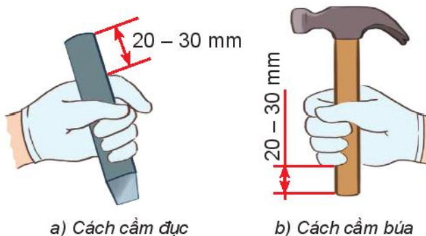
Hình 8.9. Cách cầm đục và búa
