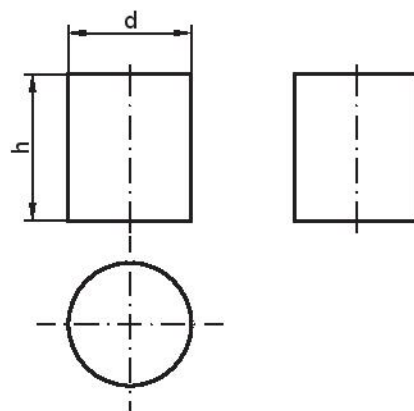
b) Các hình chiếu vuông góc
