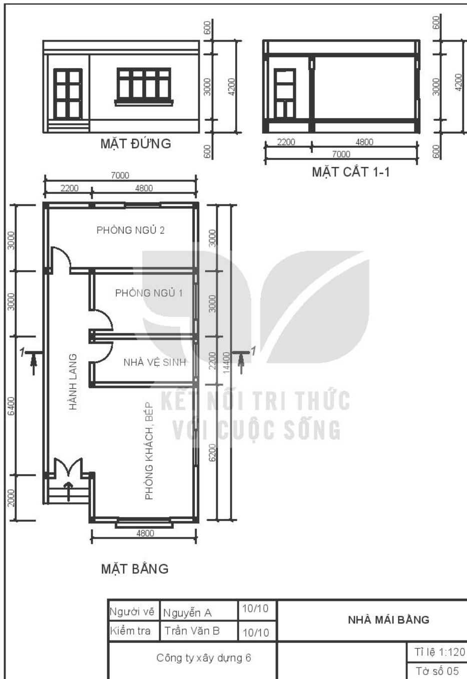
Hình 5.4. Bản vẽ ngôi nhà mái bằng
