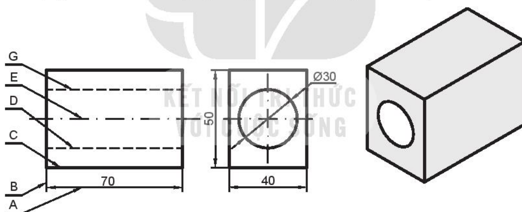
Hình 1.4. Ứng dụng các nét vẽ
