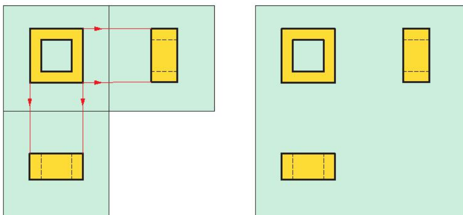
a) Các mặt phẳng hình chiếu sau khi mở
