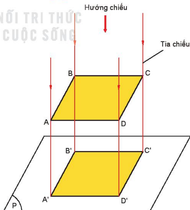
Hình 2.2. Phép chiếu vuông góc
