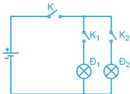
Hình 14.1. Sơ đồ mạch điện đơn giản
