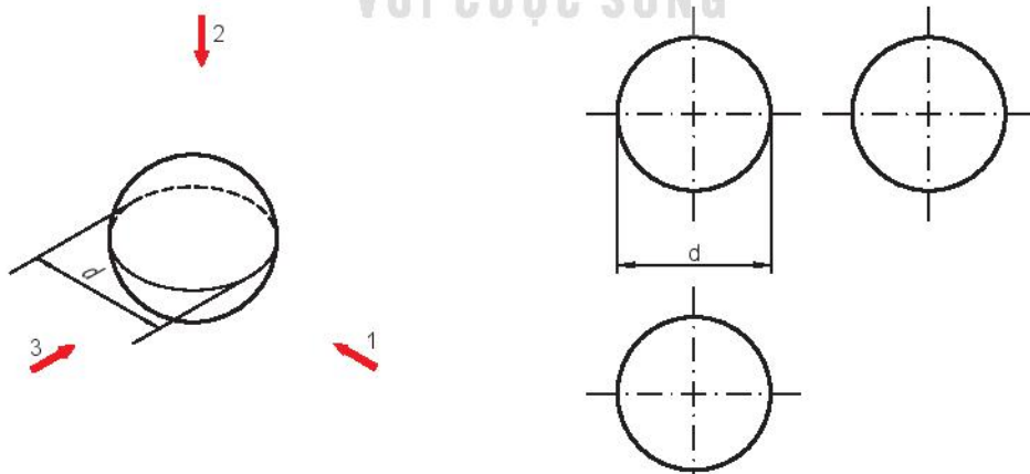
a) Hình cầu và các hướng chiếu
