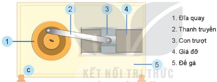
Hình 7.6. Bộ mô hình truyền và biến đổi chuyển động
