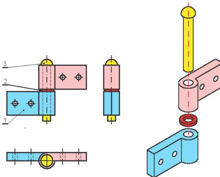
Hình 4.7. Tô màu phân biệt các chi tiết
