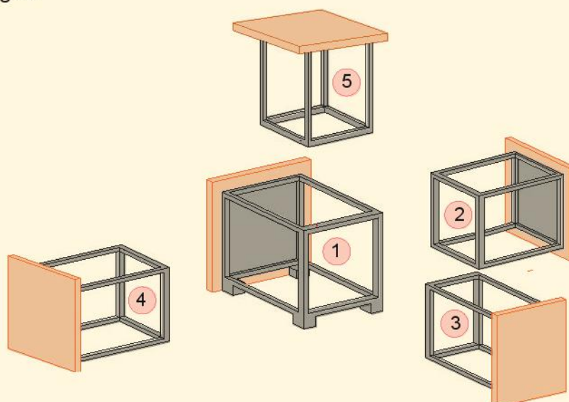
Hình 19.4. Bộ ghế lồng ghép
