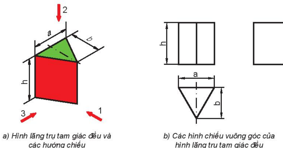
Hình 2.8. Hình lăng trụ tam giác đều và các hình chiếu vuông góc
