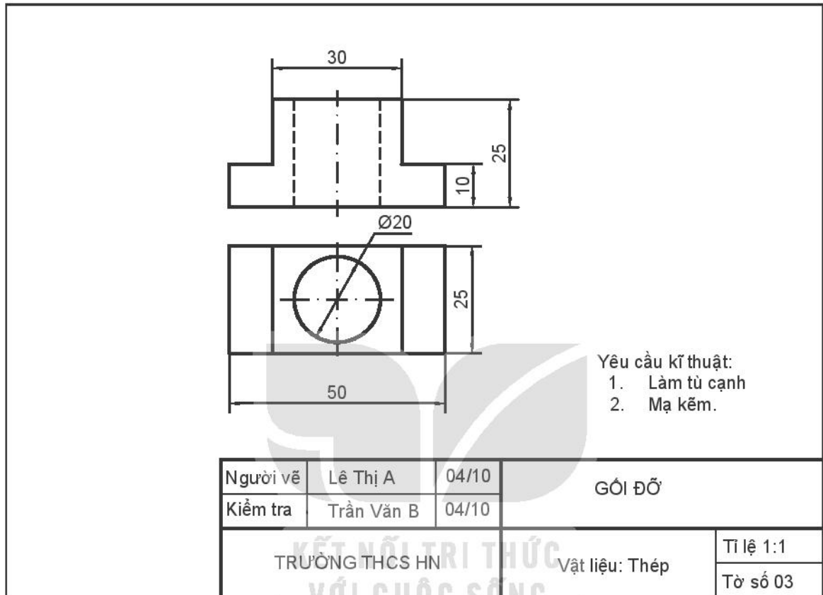
Hình 3.6. Bản vẽ gối đỡ
