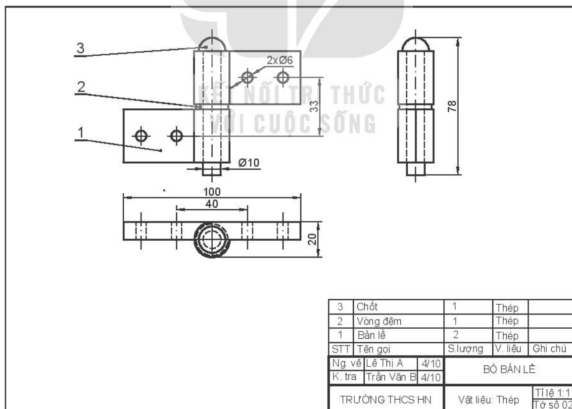
Hình 4.6. Bản vẽ lắp của bộ bản lề
