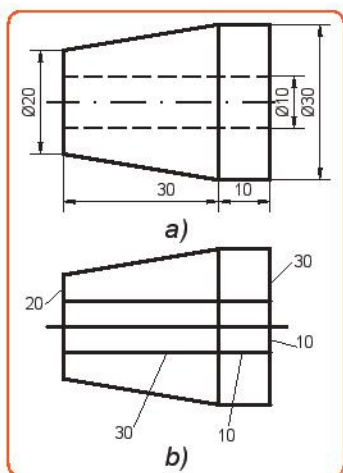
Hình 1.1. Hình biểu diễn
