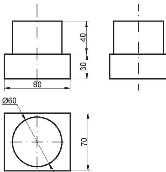
Hình 2.24. Tô nét, ghi kích thước
