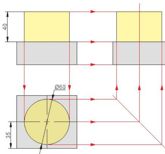
Hình 2.23. Vẽ khối trụ (2)
