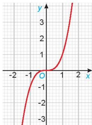
Đồ thị hàm số y = g(x) = x^3
