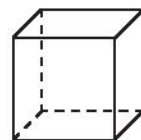
Hình 4.3. Hình biểu diễn của hình chóp tam giác đều và hình lập phương
