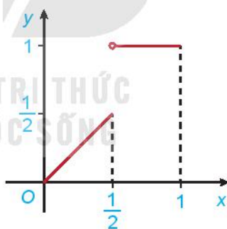
Hàm số y = g(x)
