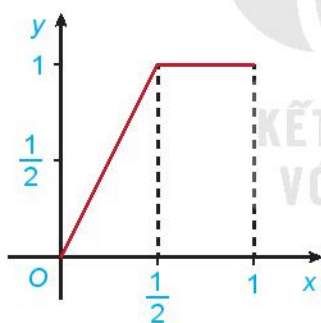
Hàm số y = f(x)
