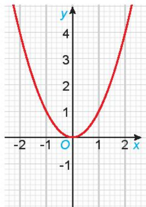
Đồ thị hàm số y = f(x) = x^2
