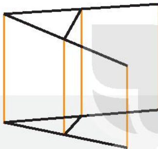
Hình chiếu của hình chữ “A”
