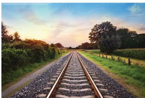
Khi nhìn hai đường ray xe lửa ta có cảm giác chúng “cắt nhau ở xa vô tận”
