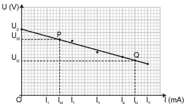
Hình 26.3. Đồ thị quan hệ U và I của pin điện hoá
