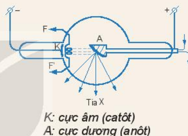
Hình 18.2. Cấu tạo ống phóng tia X
