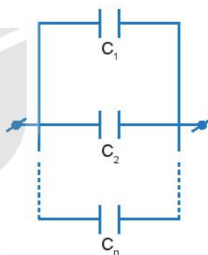
Hình 21.8. Bộ tụ điện ghép song song
