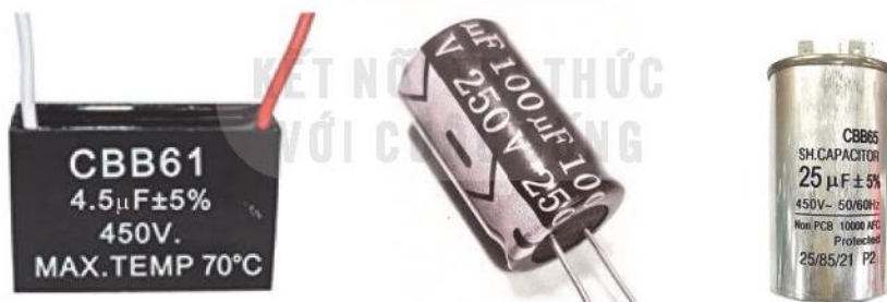
Hình 21.1. Một số loại tụ điện
