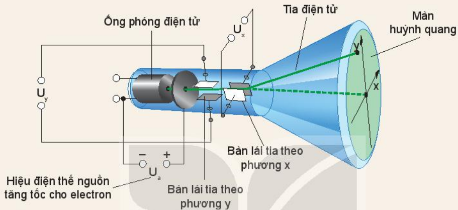
Hình 18.6. Mô hình ống phóng tia điện tử
