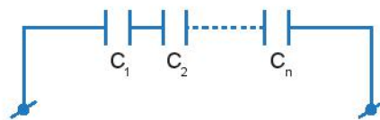
Hình 21.7. Bộ tụ điện ghép nối tiếp
