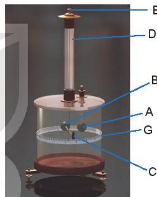
Hình 16.4. Cân xoắn Coulomb
