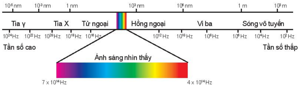
Hình 11.3. Thang sóng điện từ
