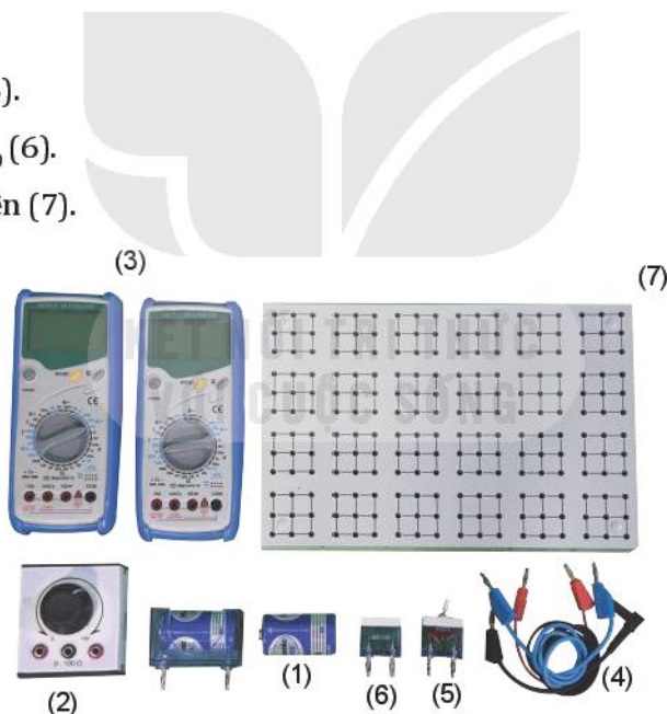
Hình 26.1. Bộ thí nghiệm đo suất điện động và điện trở trong của pin điện hoá
