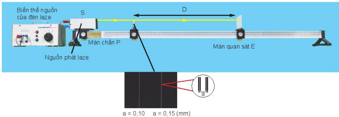
Hình 12.3. Thí nghiệm giao thoa ánh sáng
