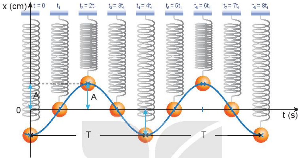
Hình 1.2. Dao động của con lắc lò xo
