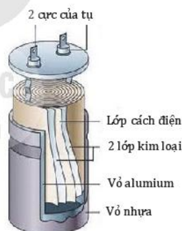
Hình 21.5. Cấu tạo của tụ điện hình trụ
