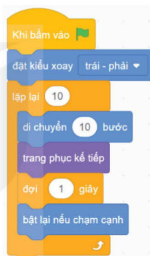
Hình 80. Chương trình vệt bay 10 lần
