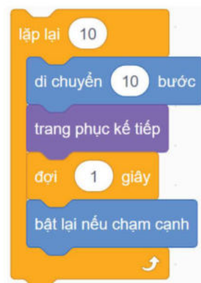
Hình 79. Khối lệnh vệt bay 10 lần
