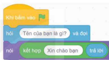
Hình 84. Chương trình "Xin chào bạn..."
