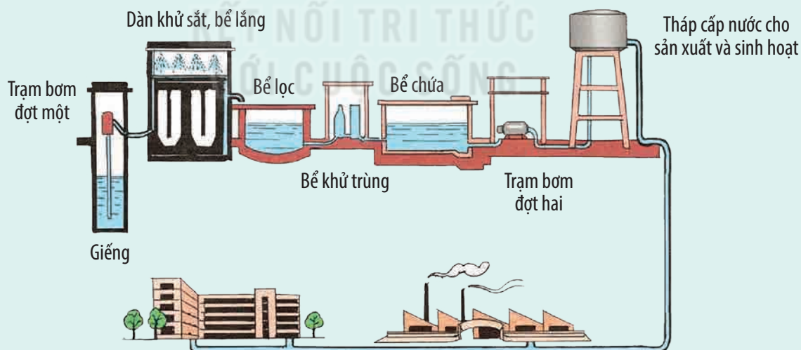
Hình 8. Sơ đồ dây chuyền sản xuất và cấp nước máy
