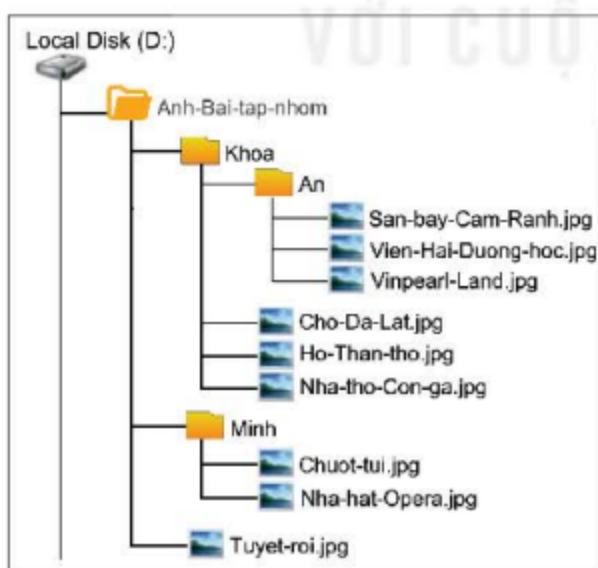
Hình 18. Cây thư mục 1
