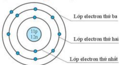
Hình 1.4. Mô hình cấu tạo nguyên tử natri
