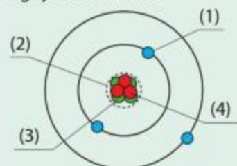
Hình 1.3. Mô hình cấu tạo nguyên tử lithium
