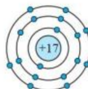
b) Chlorine
