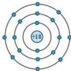
c) Argon
