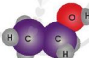
d) Ethanol
