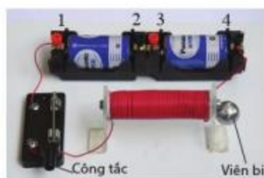
Hình 15.8. Nam châm điện đơn giản
