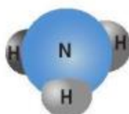
c) Ammonia
