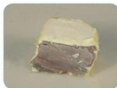
a) Natri
