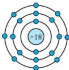
b) Argon
