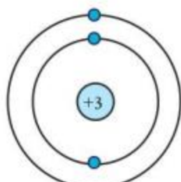
a) Lithium
