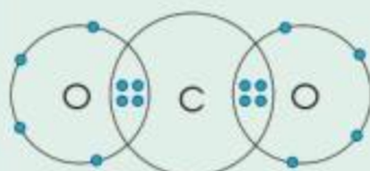
Hình 6.3. Sơ đồ liên kết cộng hoá trị giữa C và O trong phân tử khí carbonic
