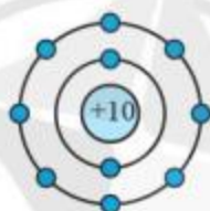
b) Neon
