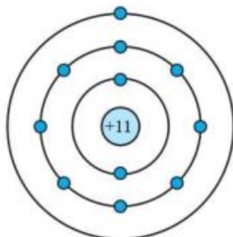
a) Natri
