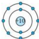
b) Neon
