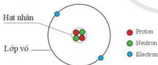
Hình 1.2. Mô hình cấu tạo nguyên tử helium
