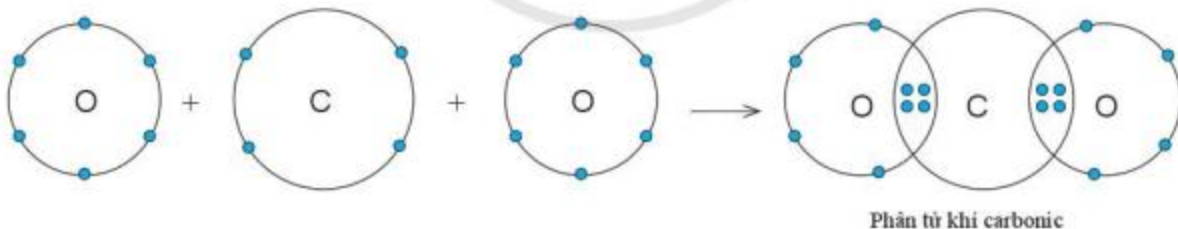
Hình 5.11*. Sơ đồ tạo thành liên kết trong phân tử khí carbonic
