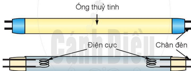
Hình 12.3. Cấu tạo của đèn huỳnh quang ống
