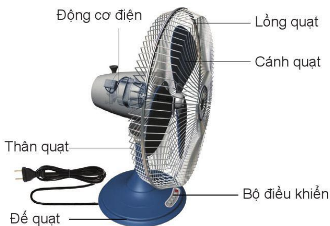
Hình 14.2. Cấu tạo của quạt điện
