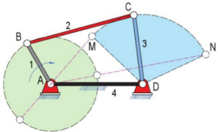
Hình 8.12. Cơ cấu tay quay thanh lắc
