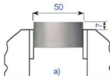
Hình 7.15. Phôi thép
