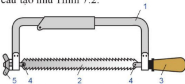
Hình 7.2. Hình dạng và cấu tạo cưa tay
