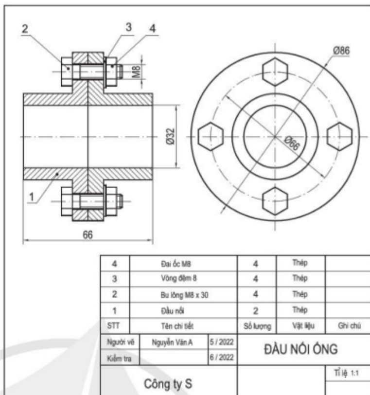
Hình 4.3. Bản vẽ lắp đầu nối ống
