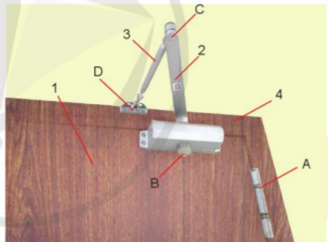
Hình 8.13. Cơ cấu đóng cửa tự động
