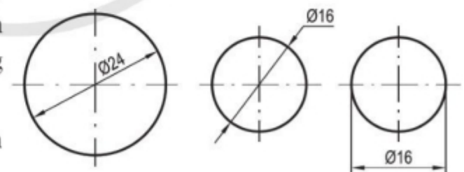
Hình 1.3. Cách ghi kích thước đường tròn
