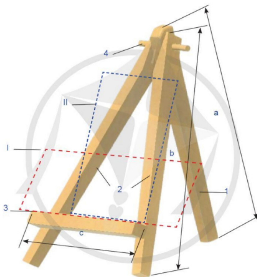
Hình 17.5. Bản vẽ mô hình giá đỡ điện thoại bằng gỗ
