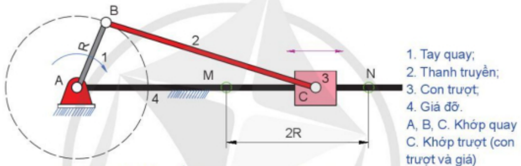
Hình 8.10. Cơ cấu tay quay con trượt
