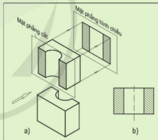
Hình 4.4. Vẽ hình cắt toàn phần
