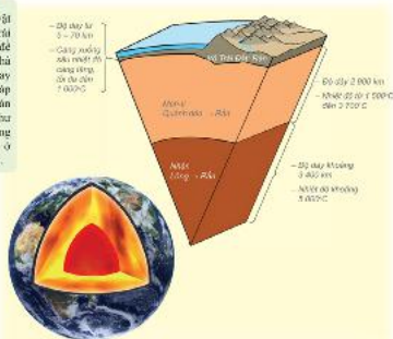
Hình 1. Cấu tạo bên trong của Trái Đất
