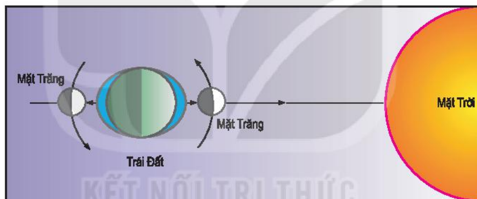
Hình 12.3. Vị trí của Mặt Trăng, Trái Đất và Mặt Trời vào các ngày “triều cường” (lực tạo triều lớn nhất)
