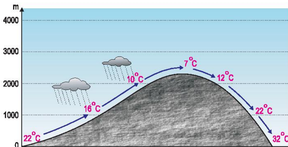
Hình 9.6. Gió fon
