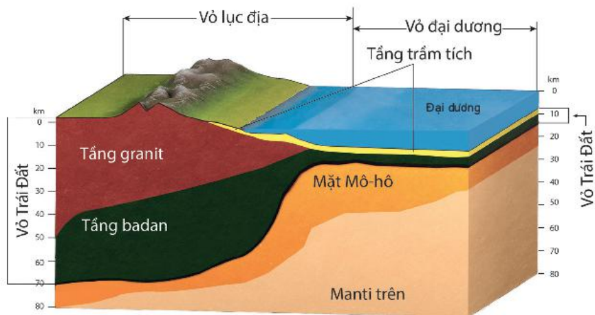
Hình 4. Sơ đồ cấu tạo vỏ Trái Đất
