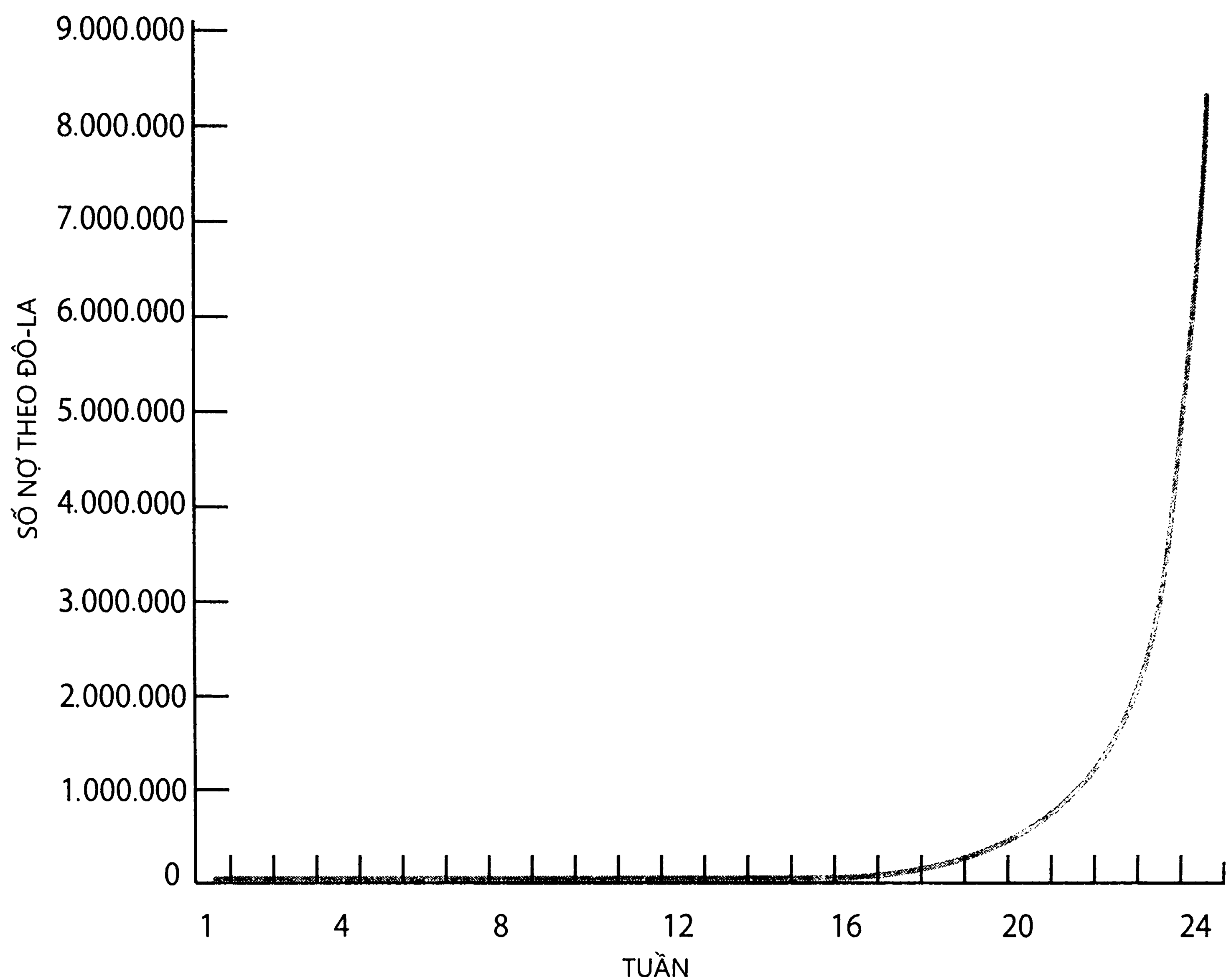
Hình 3.4. Tách cà phê trị giá 8 triệu đô-la: lãi suất tổng hợp được dựng trên đồ thị truyền thống. Mặc dù chi phí của một tách cà phê tăng dần từ 1 đô-la đến 8.192 đô-la qua 14 tuần, cuộc đua đến thảm họa tài chính vẫn chưa thấy xuất hiện trên đồ thị mãi cho đến tuần 17.
