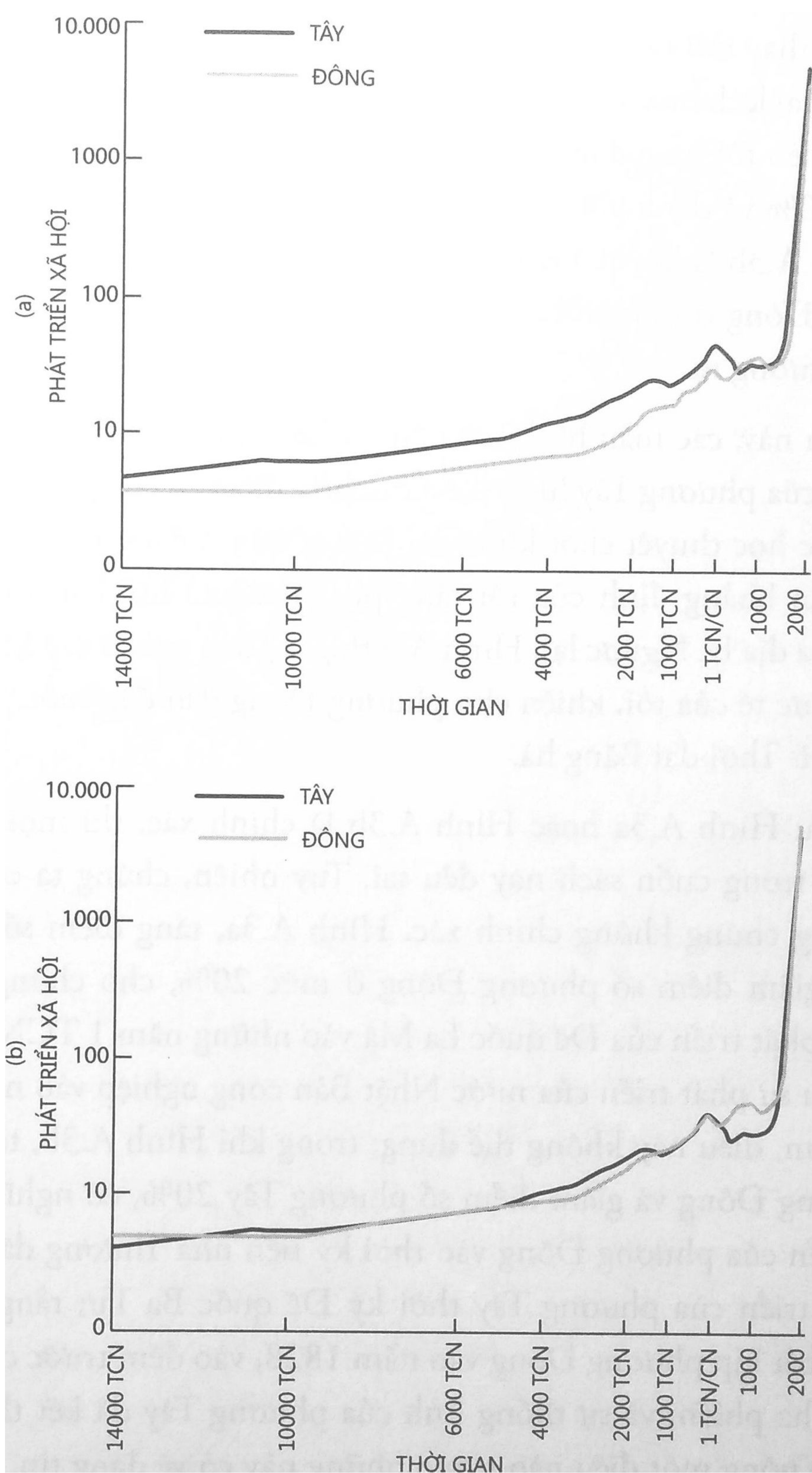
Hình A.2. Sai số được thể hiện: các hàm ý lỗi hệ thống trong điểm số phát triển xã hội. (a) tăng tất cả điểm số phương Tây lên 10% và giảm tất cả các điểm số phương Đông với tỉ lệ tương tự; (b) tăng tất cả điểm số phương Đông lên 10% và giảm tất cả điểm số phương Tây với tỉ lệ tương tự.
