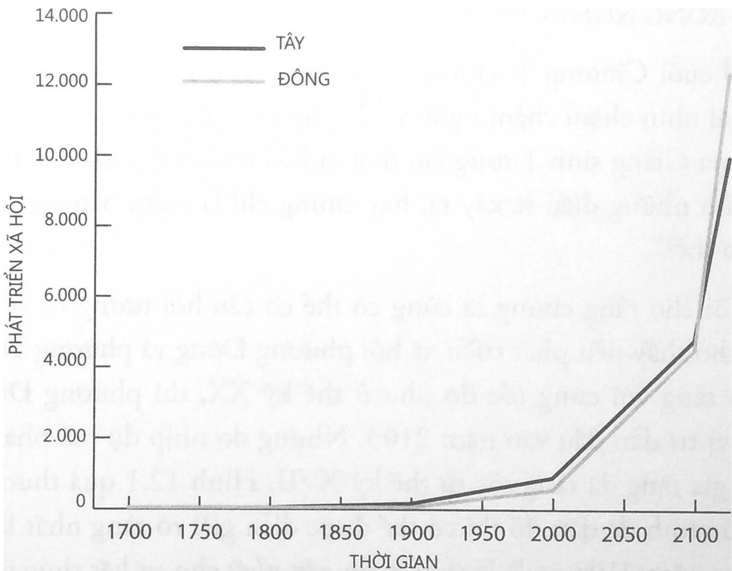
Hình 12.1. Tính toán không đối? Nếu điểm số phát triển xã hội ở phương Đông và phương Tây gia tăng cùng một tốc độ như trong thế kỷ XX, thì sự dẫn đầu của phương Tây sẽ kết thúc vào năm 2103.
