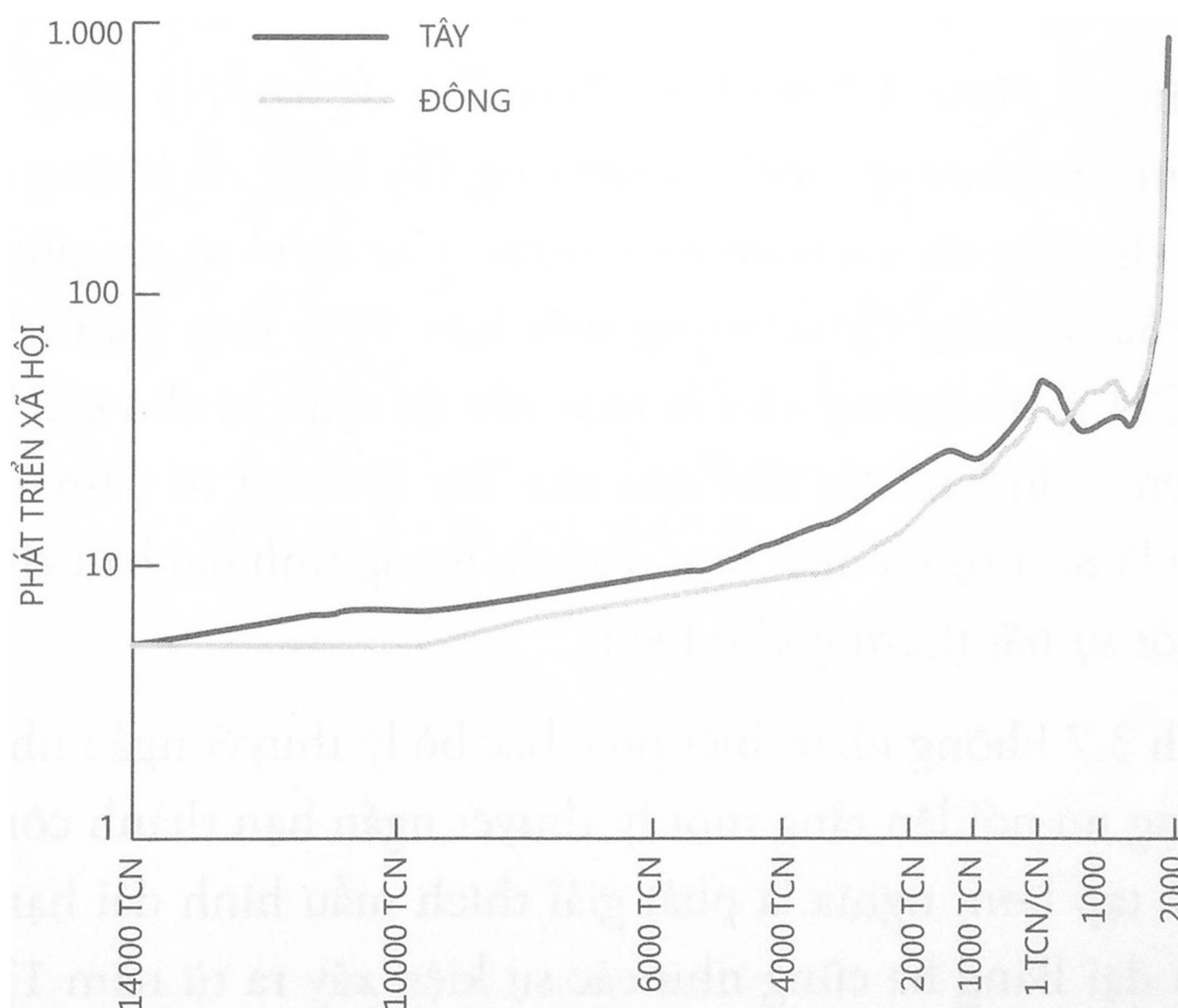
Hình 3.7. Sự tăng trưởng của phát triển xã hội, năm 14000 TCN-2000, được vẽ trên một mô hình tuyến tính Logarit. Đây có thể là cách hữu ích nhất để trình bày điểm số, làm nổi bật tỉ lệ tăng trưởng tương đối ở phương Đông và phương Tây cùng tầm quan trọng của hàng nghìn năm thay đổi trước năm 1800.
