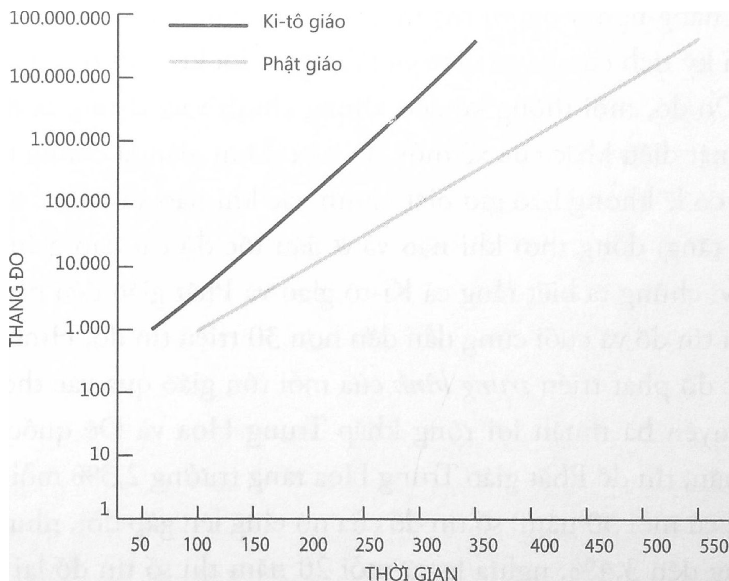
Hình 6.9. Thống kê tín đồ: Sự phát triển của Ki-tô giáo và Phật giáo Trung Hoa, giả định rằng các tỉ lệ thay đổi bất biến. Tỉ lệ dọc tính theo logaríi, như trong Hình 3.6 và 3.7, do đó tỉ lệ tăng trưởng trung bình bất biến (3,4% mỗi năm đối với Ki-tô giáo, 2,3% đối với Phật giáo) tạo ra các đường thẳng.
