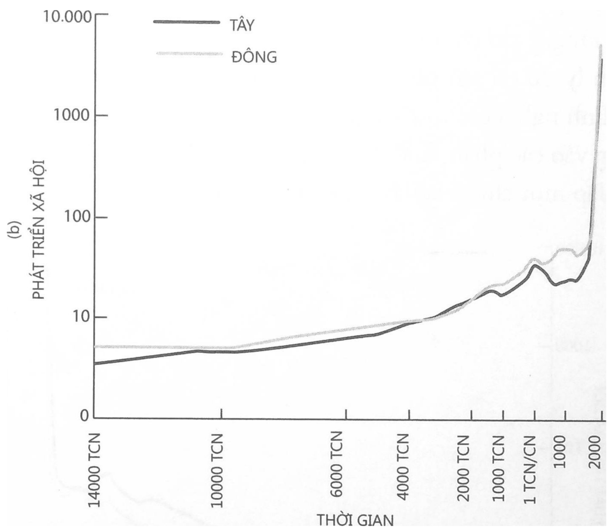
Hình A.3. Sai số thậm chí lớn hơn: (a) tăng tất cả điểm số phương Tây và giảm tất cả điểm số phương Đông ở mức 20%, và (b) tăng tất cả điểm số phương Đông và giảm tất cả điểm số phương Tây ở mức 20%.
