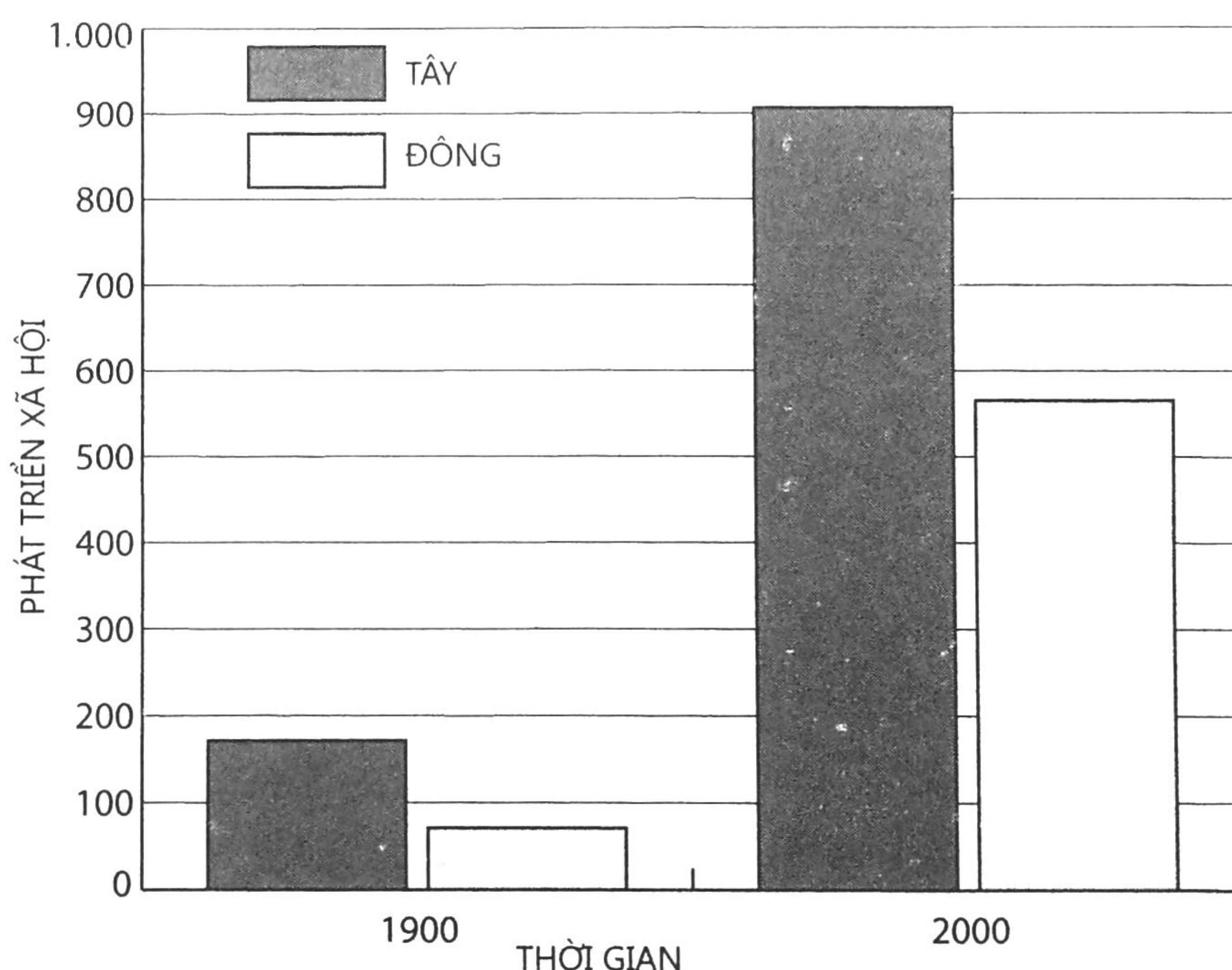
Hình 10.11. Biết ngọn gió đổi theo chiều nào: Thế kỷ XX có phải là điểm đỉnh đồng thời là điểm kết thúc sự thống lĩnh của phương Tây? Sự dẫn đầu của phương Tây trong phát triển xã hội đã tăng từ 101 điểm năm 1900 lên 336 điểm vào năm 2000, nhưng tỉ lệ điểm số giữa phương Tây và phương Đông rút xuống 1/3, từ 2,4/1 vào năm 1900 xuống còn 1,6/1 vào năm 2000.
