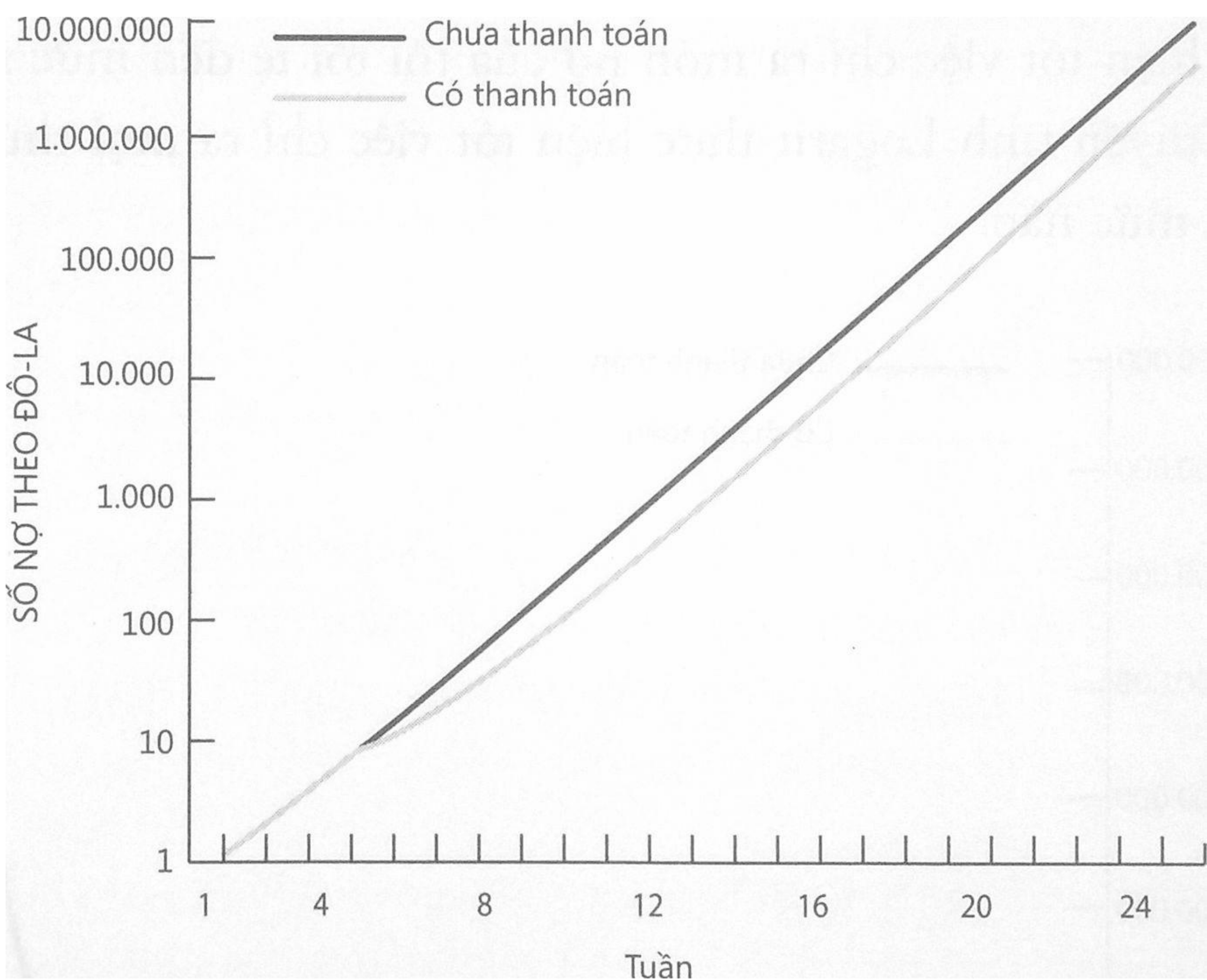
Hình 3.6. Con đường thẳng dẫn đến thảm họa: vòng xoáy của món nợ trên một quy mô logic tuyến tính. Đường màu đen biểu thị số nợ tăng gấp đôi nếu không thanh toán, trong khi đường màu xám cho thấy tác động của các khoản thanh toán nhỏ lẻ từ tuần 5 đến tuần 9 trước khi nó tăng gấp đôi khi ngừng các khoản thanh toán.
