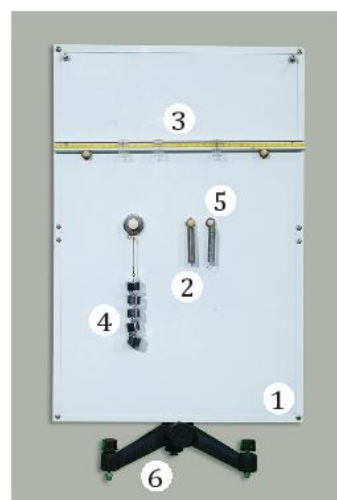
Hình 22.3. Bộ thí nghiệm tổng hợp hai lực song song cùng chiều
