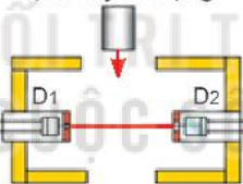
Hình 6.1. Cấu tạo cổng quang điện
