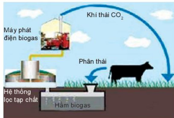
Hình 10.3. Chu trình sản xuất bioga
