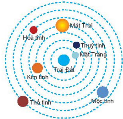
Hình 5.13. Mô hình hệ địa tâm của Ptolemy
