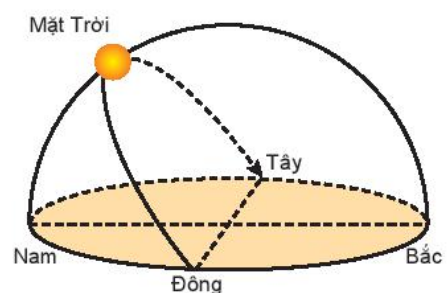
Hình 5.4. Mặt Trời mọc và lặn
