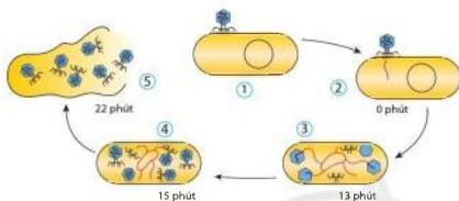
Hình 21.4. Sơ đồ các giai đoạn trong chu trình nhân lên của phage T4 gây bệnh lỵ vi khuẩn E. coli
