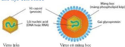
Hình 21.2. Các thành phần cấu tạo virus
