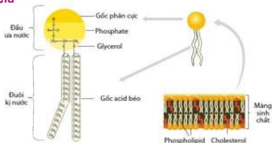
Hình 6.11. Phospholipid cấu tạo nên màng sinh chất
