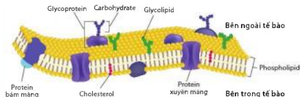
Hình 8.2. Cấu trúc của màng sinh chất
