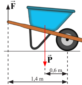
▲ Hình 14.11. Xe đẩy vật liệu
