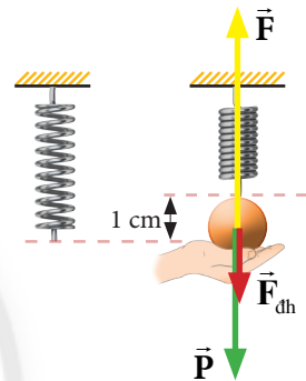
▲ Hình 23.5. Lực tác dụng lên vật để lò xo bị nén
