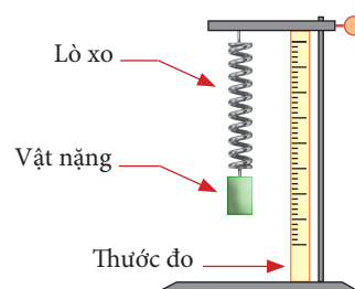
▲ Hình 23.1. Sơ đồ bố trí thí nghiệm
