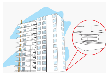
▲ Hình 22.7. Lò xo được đặt dưới móng cọc nhà cao tầng ở Nhật Bản
