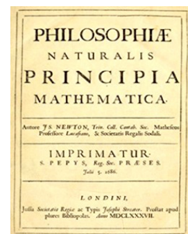
▲ Hình 10.5. Một ấn bản của tác phẩm trong đó Newton trình bày các định luật về chuyển động
