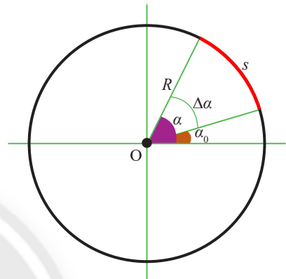
Hình 20.7. Độ dịch chuyển góc \Delta\alpha
