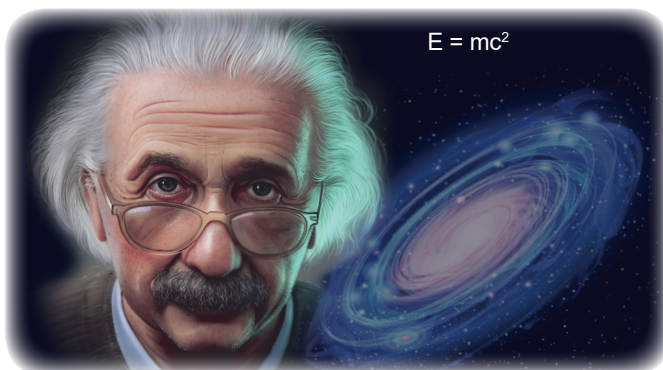
▲ Hình 1.1. Albert Einstein (1879 – 1955)
