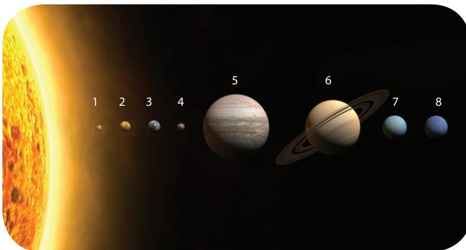
▲ Hình 1.4. Mô hình mô phỏng vị trí các hành tinh trong hệ Mặt Trời: 1. Thủy tinh; 2. Kim tinh; 3. Trái Đất; 4. Hoả tinh; 5. Mộc tinh; 6. Thổ tinh; 7. Thiên Vương tinh; 8. Hải Vương tinh
