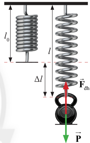
▲ Hình 23.3. Lò xo bị dãn khi treo vật vào
