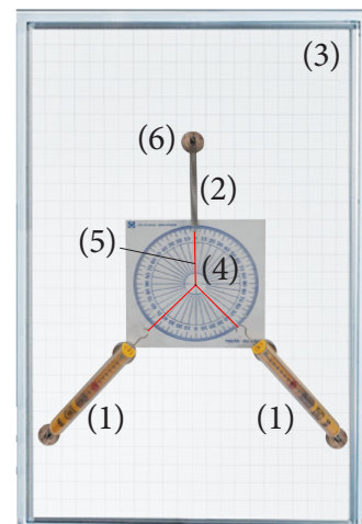
▲ Hình 13.11. Gợi ý bố trí thí nghiệm
