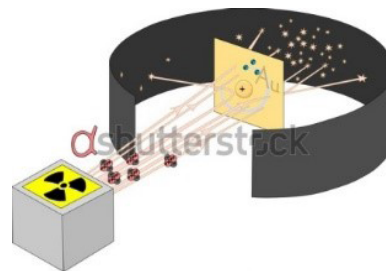
▲ Hình 1P.1. Thí nghiệm Rutherford
