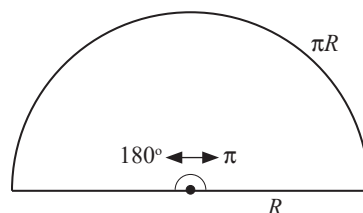
▲ Hình 20.4. Minh họa góc \pi rad
