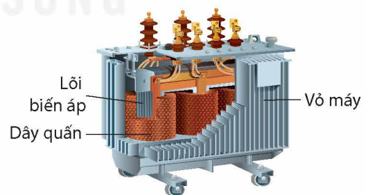
Hình 3.2. Mô tả một số bộ phận của máy biến áp
