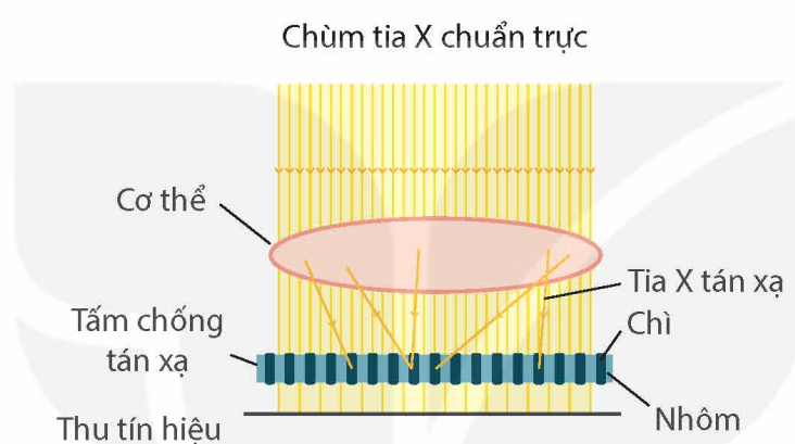
Hình 6.7. Sơ đồ minh họa các tia X tán xạ bị hấp thụ bởi tấm chống tán xạ
