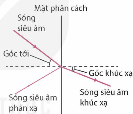
Hình 7.3. Một sóng siêu âm khi chạm vào ranh giới giữa hai vật liệu khác nhau, vừa bị khúc xạ vừa bị phản xạ
