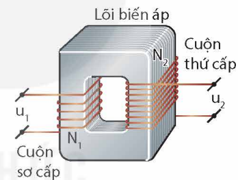
Hình 3.1. Sơ đồ cấu tạo chính của máy biến áp
