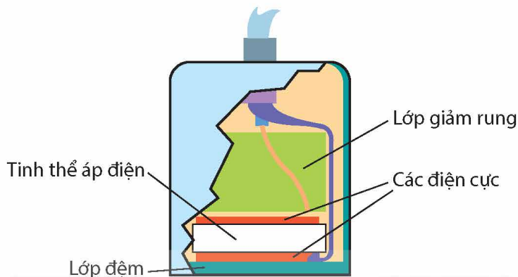
Hình 7.2. Cấu tạo của đầu dò siêu âm
