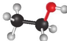
a) Mô hình quả cầu – thanh nối b) Mô hình đặc
