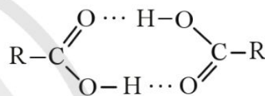
b) Dạng dimer vòng
