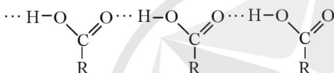
a) Dạng polymer
