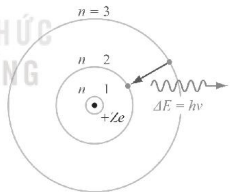
Hình 1.1. Mô hình nguyên tử theo Niels Bohr
