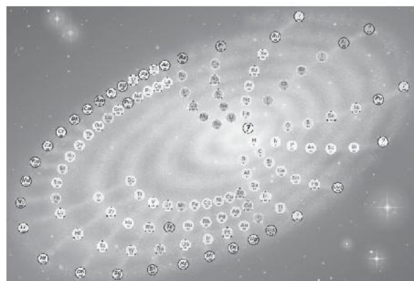
Hình 5.5. Thiên hà nguyên tố của Philip Stewart (2004)
