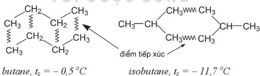
Hình 13.4. Mô tả tương tác van der Waals của butane và isobutane
