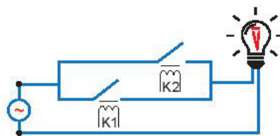
Hình 4.5. Mạch điện thực hiện phép cộng logic
