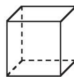
Hình 4.3. Hình biểu diễn của hình chóp tam giác đều và hình lập phương
