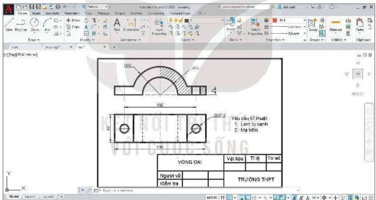
Hình 1.4. Bản vẽ kỹ thuật được vẽ bằng AutoCAD
