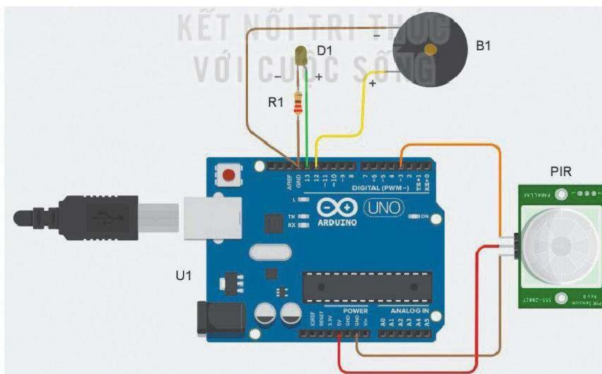
Hình 6.4. Sơ đồ nối linh kiện
