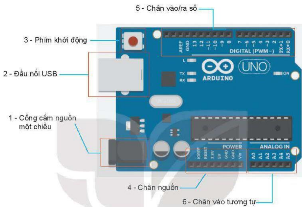
Hình 6.2. Mô tả các cổng cắm dây cáp và chân vào/ra của bảng mạch điều khiển Arduino Uno
