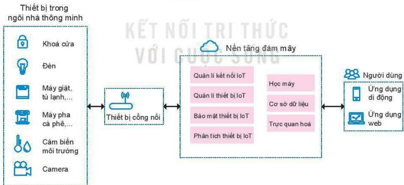
Hình 4.4. Sơ đồ khối hệ thống điều khiển cho ngôi nhà thông minh dựa trên công nghệ IoT
